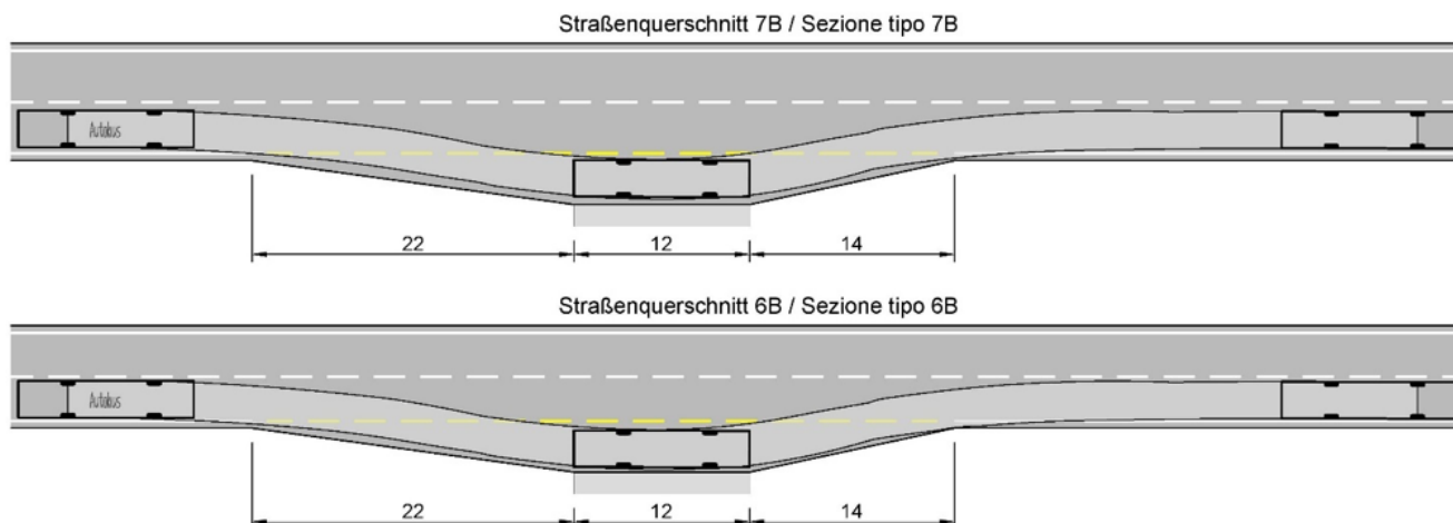
Bild B-4 Überprüfung mit den Schleppkurven der parallelen Annäherung des Busses an den Wartebereich Fig. B-4 Verifica con le curve di trascinamento dell'avvicinamento parallelo del bus all'area di attesa
