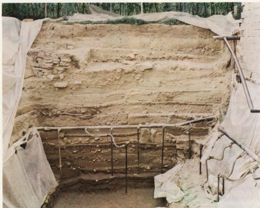
La successione degli strati nello scavo di Laimburg (parete ovest).
