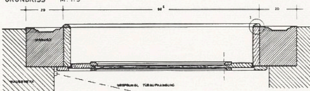
GRUNDRISS M:1:5
