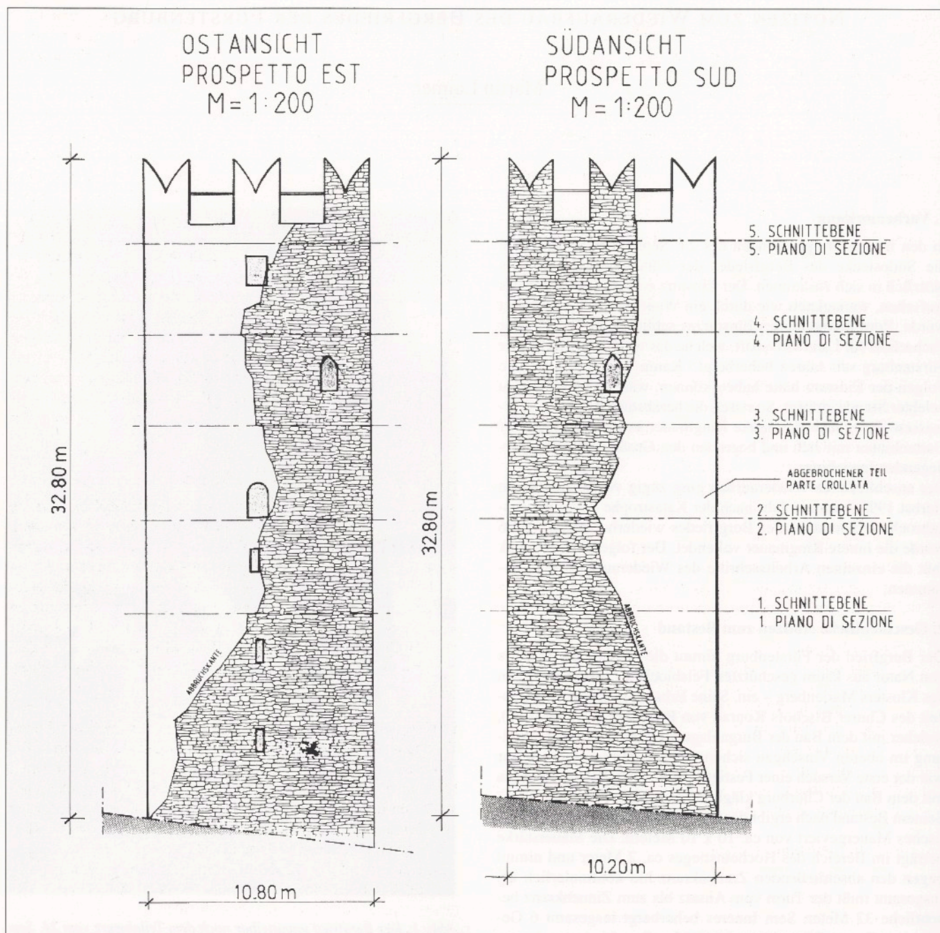
Abb. 2: Graphische Darstellung der Süd- und Ostwand nach dem Absturz
