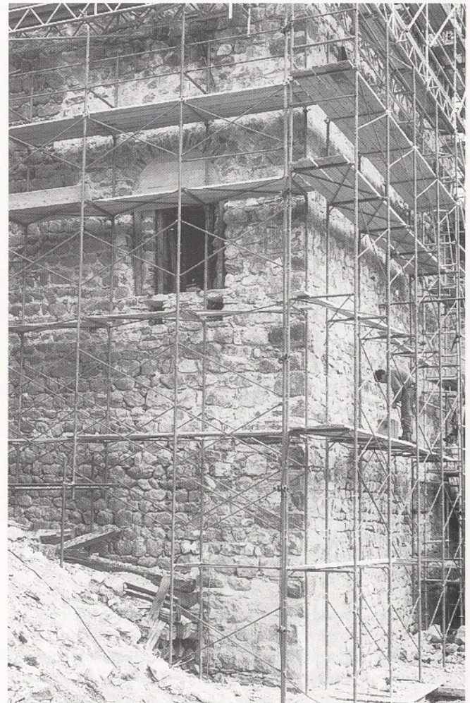
Abb. 4: Ansicht der Südostecke nach dem Wiederaufbau. Der ehemalige Hocheinstieg wurde rekonstruiert.
