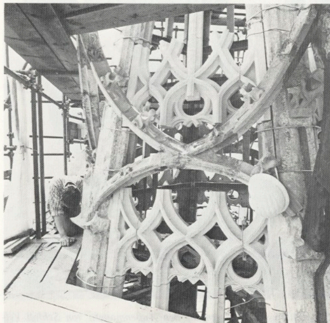
Esempio di restauro della pietra: il campanile del duomo di Bolzano. Per il momento si tratta del lavoro più impegnativo mai intrapreso dalla tutela monumentale in Alto Adige. Per la maggior parte è ormai solamente possibile la sostituzione delle singole pietre, che se per secoli hanno resistito alle intemperie, ultimamente non hanno saputo resistere all'inquinamento da acidi solforici. La struttura originale in arenaria viene per quanto possibile conservata.
