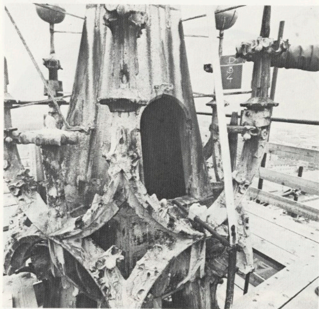
Steinrestaurierung am Beispiel des Bozner Pfarrturmes. Dieses zur Zeit aufwendige Unternehmen der Denkmalpflege in Südtirol erlaubt in großen Teilen nur mehr das Austauschen der behauenen Steine, die wohl jahrhundertlang dem Wetter, nicht mehr aber den Schwefelgasen standgehalten haben. So weit als möglich wird der Originalbestand erhalten (Sandstein).
