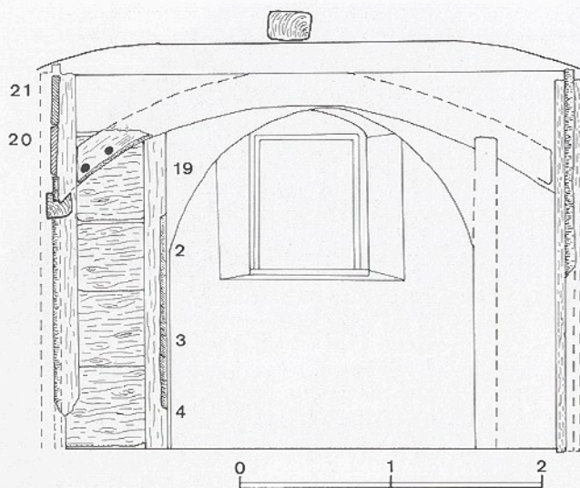
Plan der Nordwand zum Erker. Erhalten sind Teile der Eckpfosten und links die Bretter der Verkleidung und ein kleiner Teil des Stirnbrettes. Der Rest ließ sich als Abklatsch auf der Mauer nachzeichnen.
