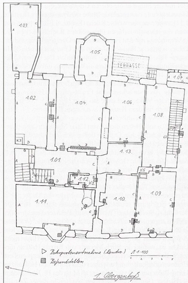
Abb. 3: Erstes Obergeschoß.
