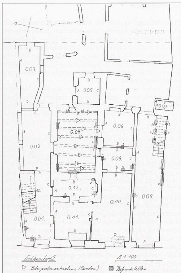
Abb. 2: Erdgeschoß.
