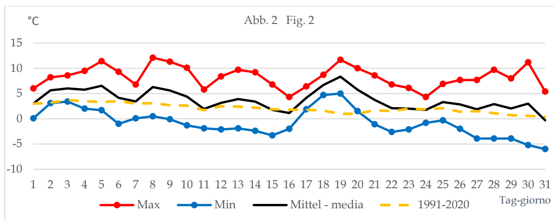
Abb. 2: Station Bozen. Tägliche Temperaturminimum (blau), -maximum (rot), Tagesmitteltemperatur (schwarz) und langjährige Tagesmitteltemperatur 1991-2020 (strichliert): Die Temperaturen lagen meist durchgehend oberhalb des Durchschnitts, erst zum Jahreswechsel wurde es spürbar kälter.
