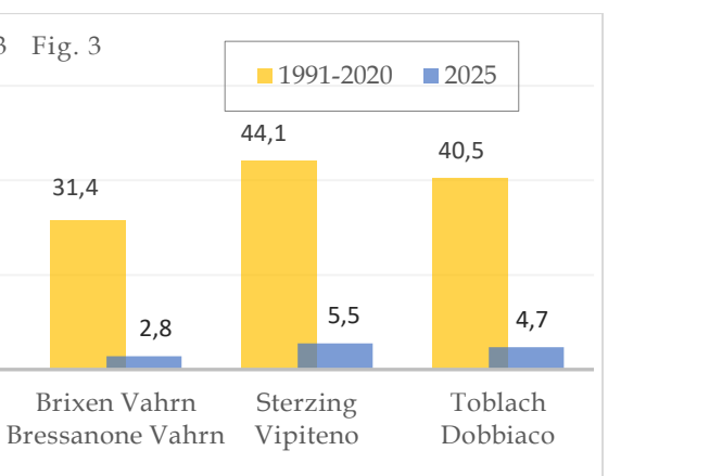
Fig. 3: precipitazione totale del mese (blu) e valori di riferimento nel periodo 1991-2020 (giallo): precipitazioni piovose e nevose quasi assenti; un momento meteorologico di rilievo è comunque la debole nevicata nelle vallate più in quota puntualmente il 24 dicembre.
