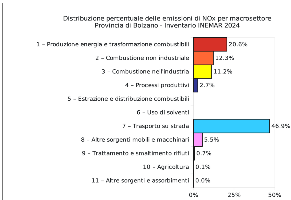
Figura 3: Distribuzione percentuale delle emissioni di NO x per tipo di fonte (anno 2024)
