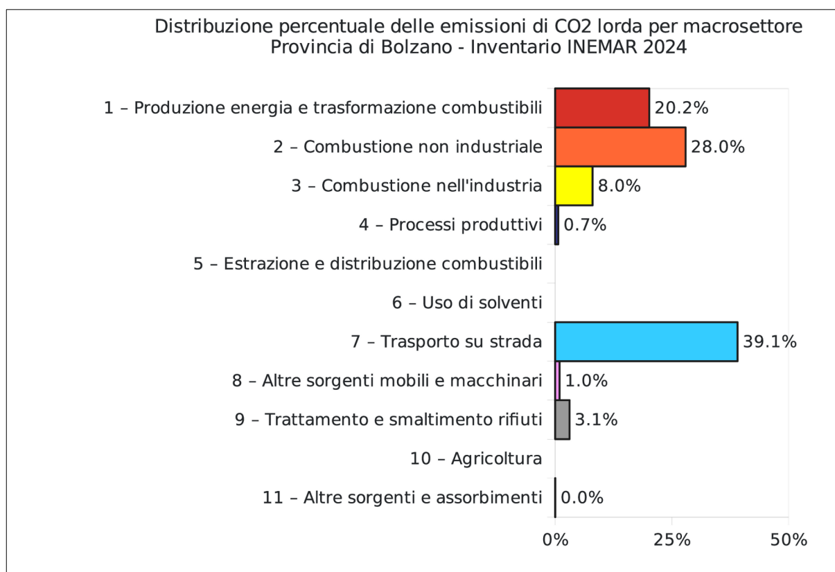
Figura 13: Distribuzione percentuale delle emissioni di CO 2 lorda per per tipo di fonte (anno 2024). Nel grafico non sono riportati gli assorbimenti della CO 2 .
