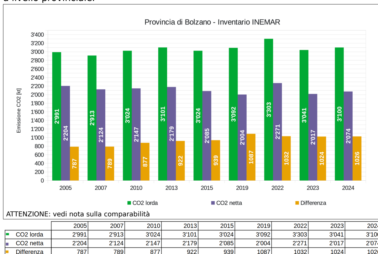
Figura 20 - Andamento delle emissioni di CO 2 Netta e Lorda negli anni 2005, 2007, 2010, 2013, 2015, 2019, 2022, 2023 e 2024.
