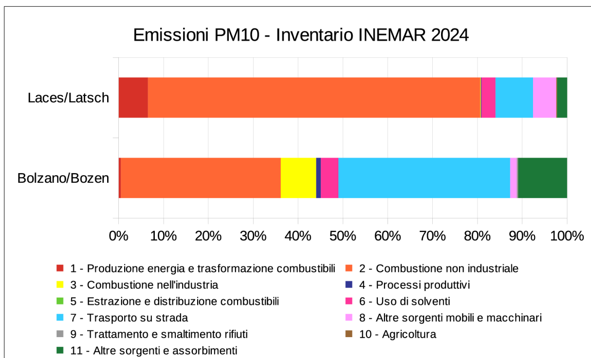
Figura 9 - Confronto emissioni di PM10 per tipo di fonte nei Comuni di Bolzano e Laces (anno 2024)
