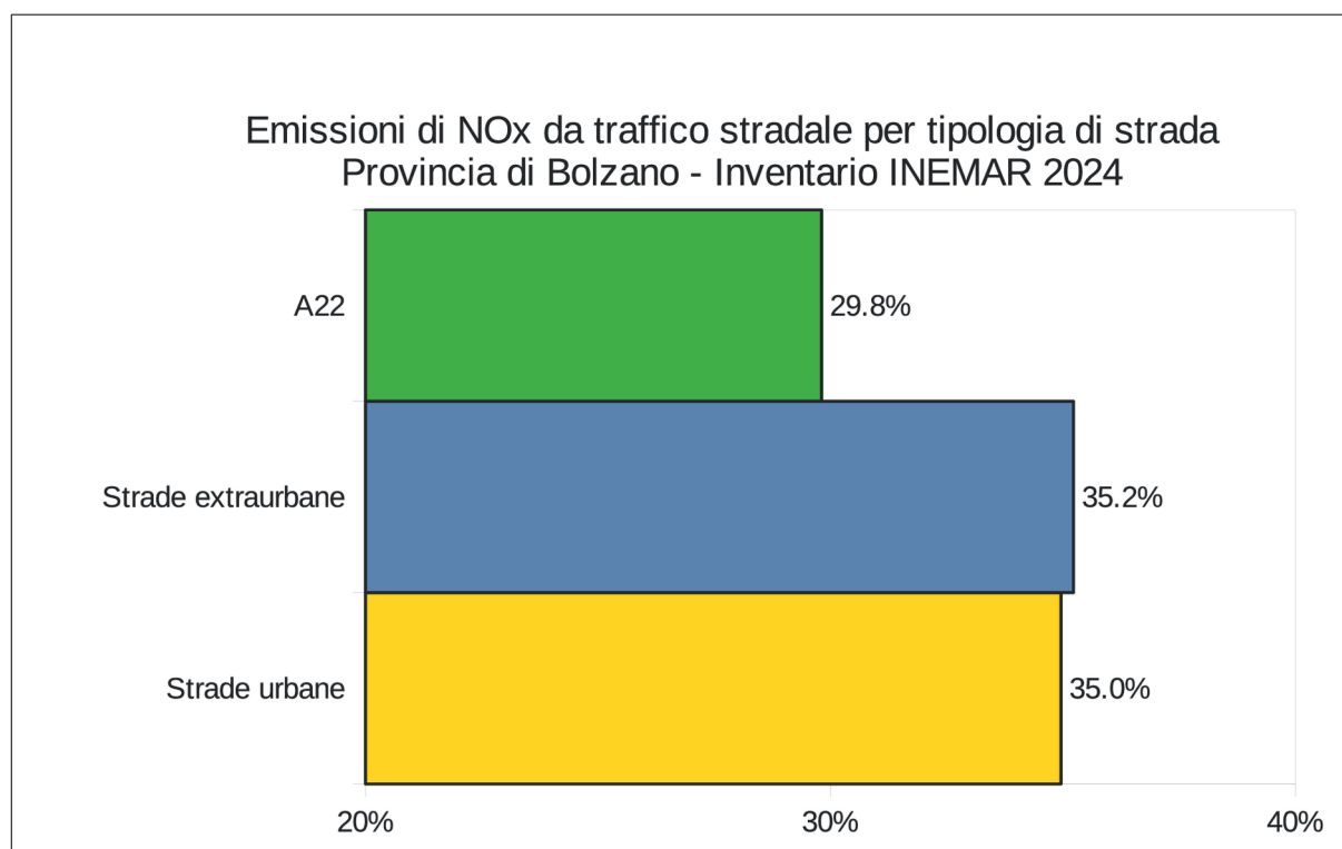
Figura 5: Quota percentuale di emissioni di NO x da traffico per tipologia di strada in Alto Adige (anno 2024)
