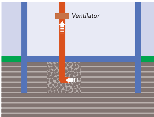
Punktuelle Unterboden-Absaugung mit Abluft über Dach.
