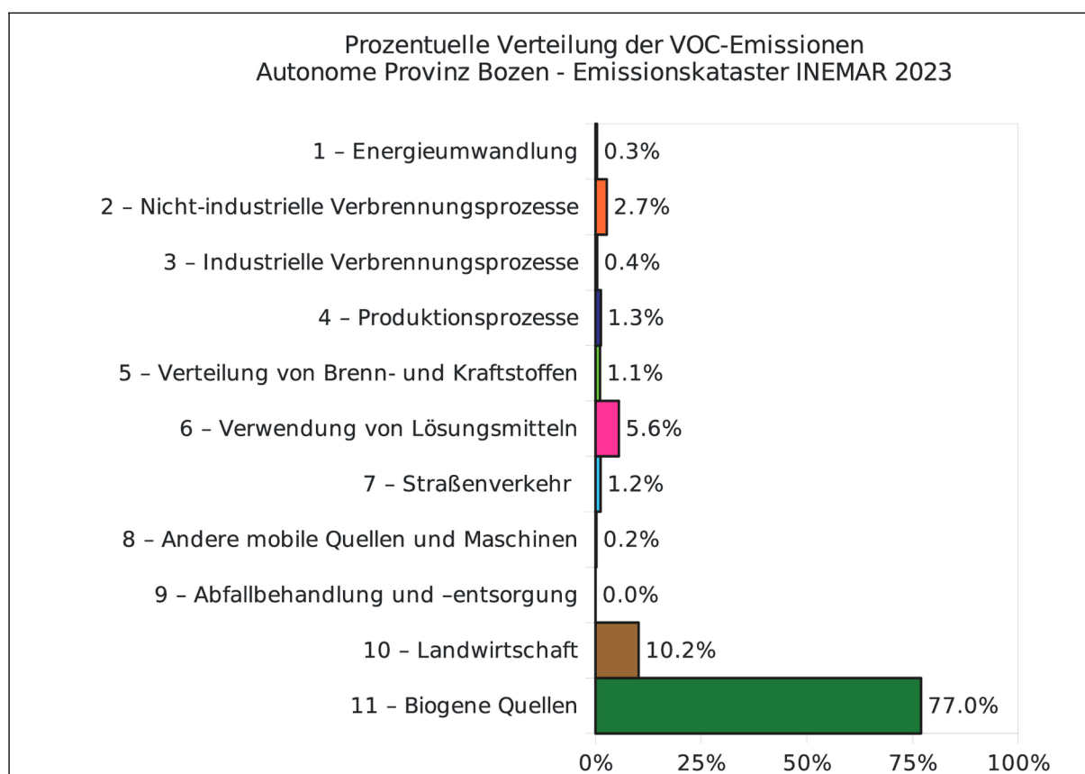
Abbildung 11: Prozentuelle Verteilung der VOC-Emissionen (Jahr 2023)
