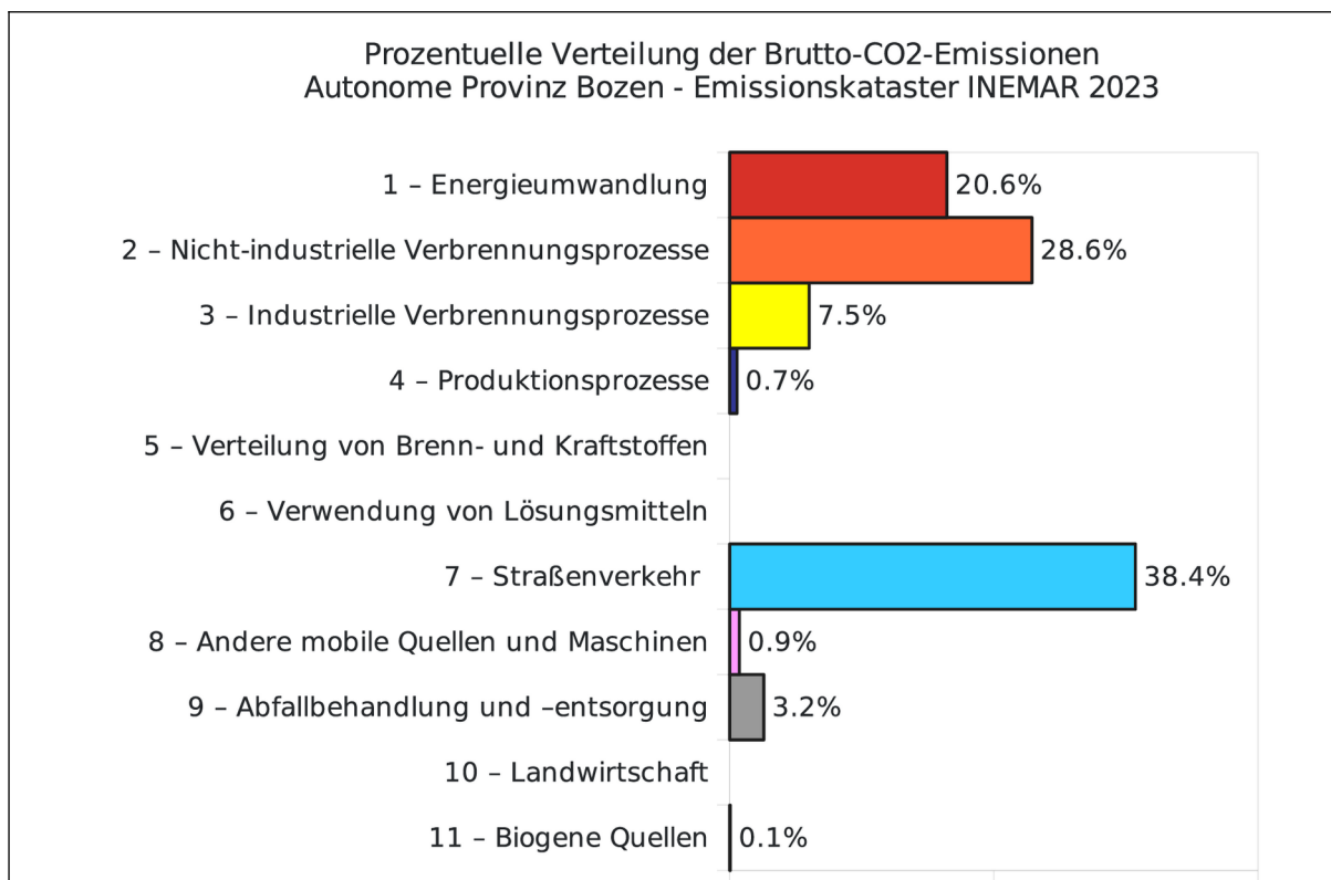
Abbildung 13: Prozentuelle Verteilung der Brutto-CO 2 -Emissionen (2023). Das in der Grafik dargestellte CO 2 berücksichtigt nicht die Absorption.
