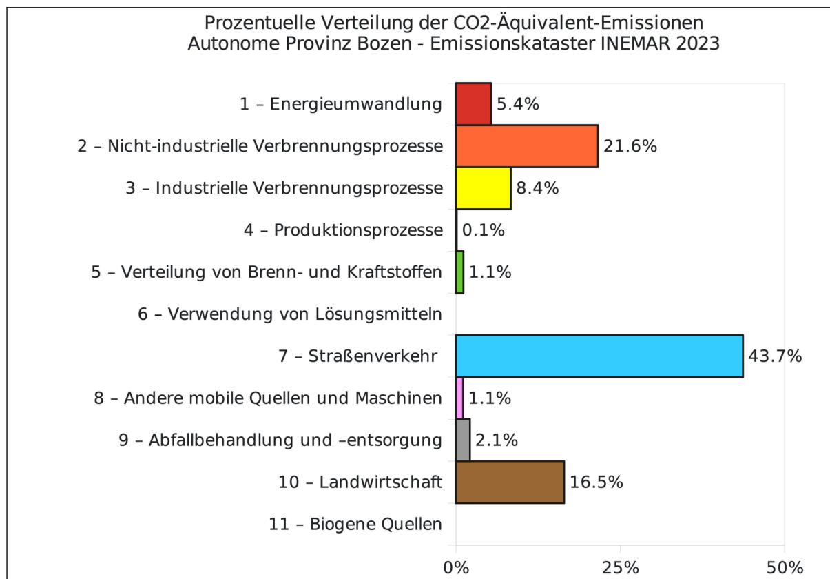
Abbildung 19: Prozentuelle Verteilung der CO 2 -Äquivalent-Emissionen (Jahr 2023). Das in der Grafik dargestellte CO 2 berücksichtigt nicht die Absorption.
