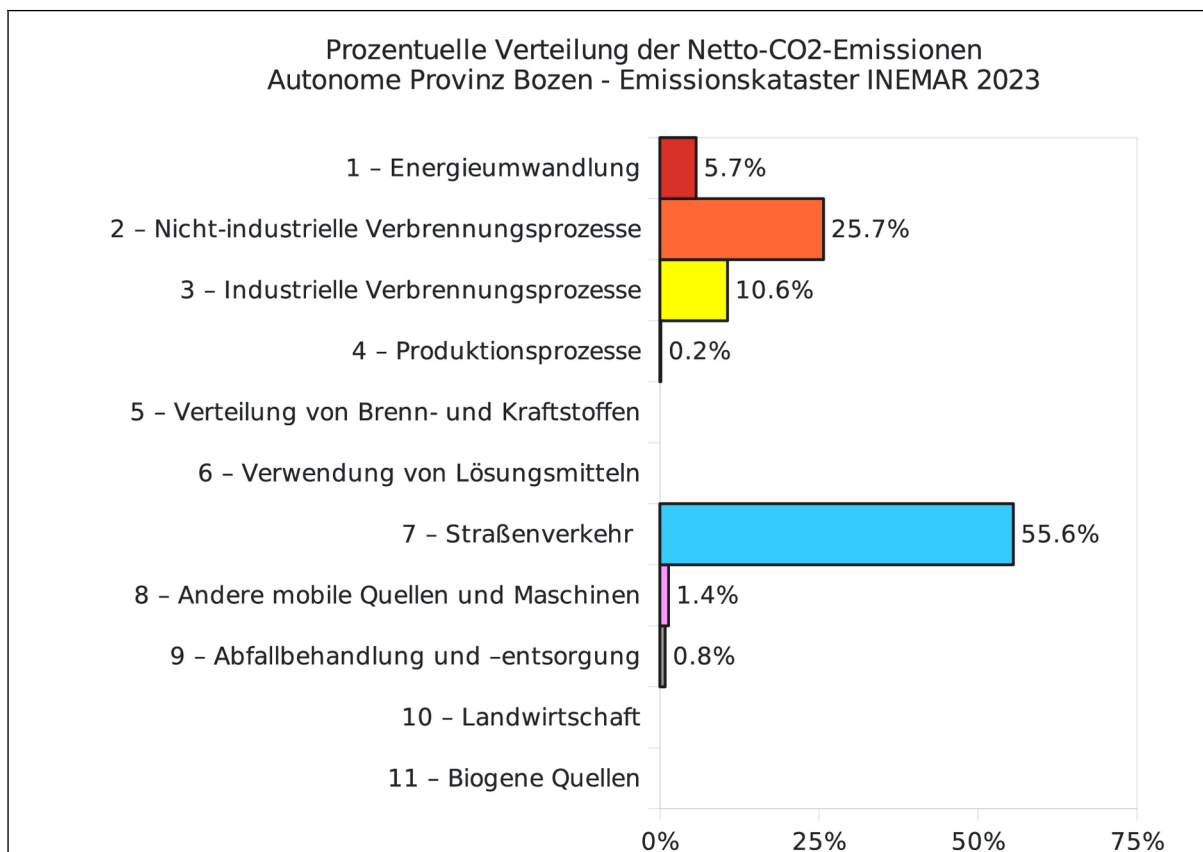
Abbildung 14: Prozentuelle Verteilung der Netto-CO 2 -Emissionen (2023). Das in der Grafik dargestellte CO 2 berücksichtigt nicht die Absorption.
