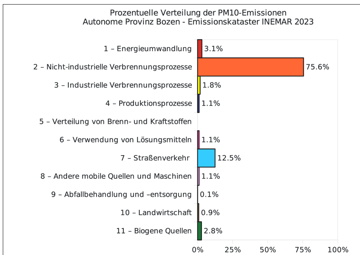
Abbildung 7: Prozentuelle Verteilung der PM10-Emissionen (Jahr 2023)
