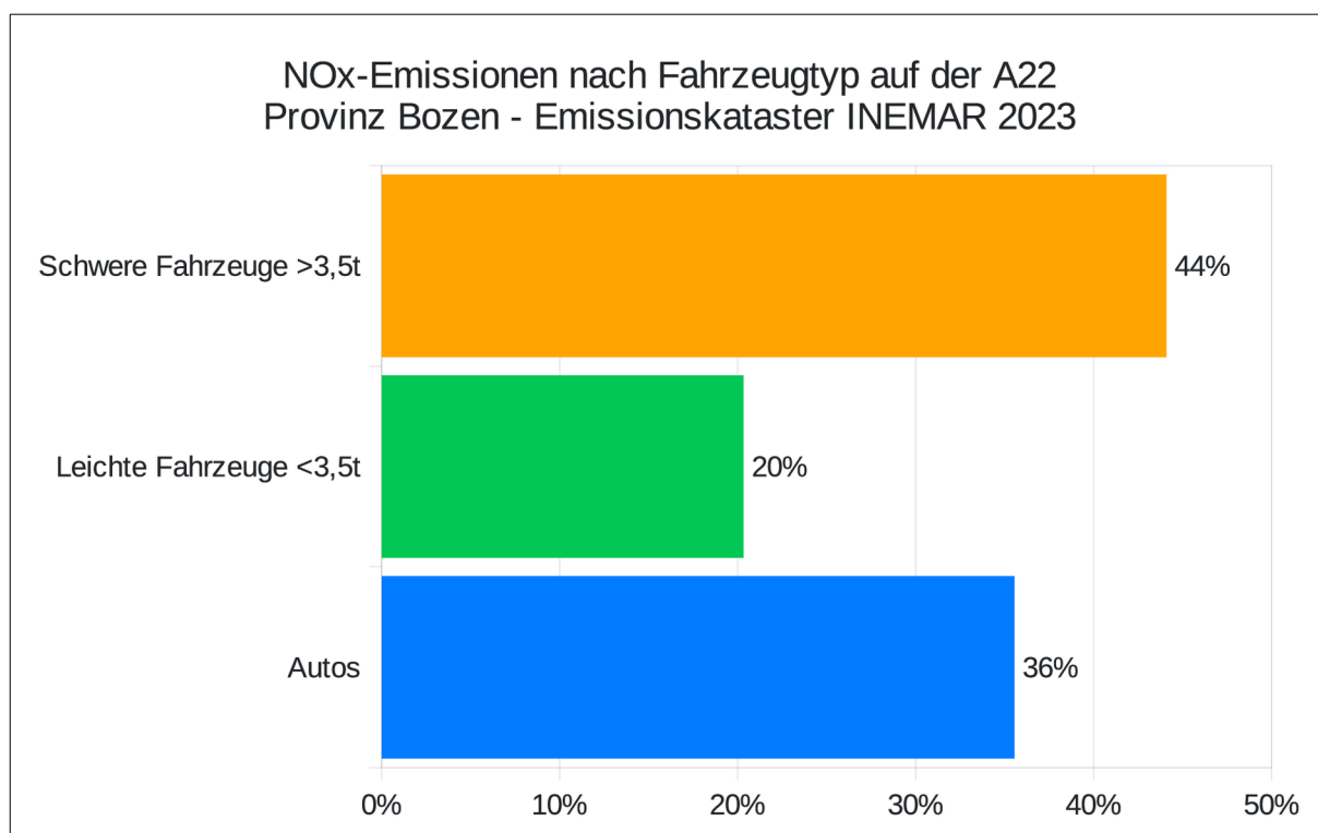
Abbildung 4: Anteil unterschiedlicher Fahrzeugtypen an der NO x Emission der A22 (Jahr 2023)
