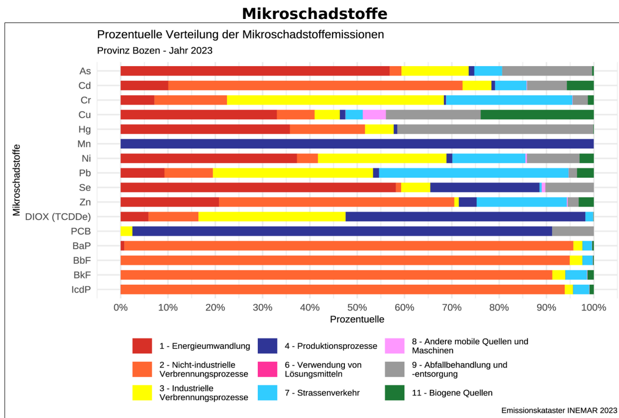
Abbildung 2: Prozentuelle Verteilung der Mikroschadstoffemissionen im Jahre 2023
