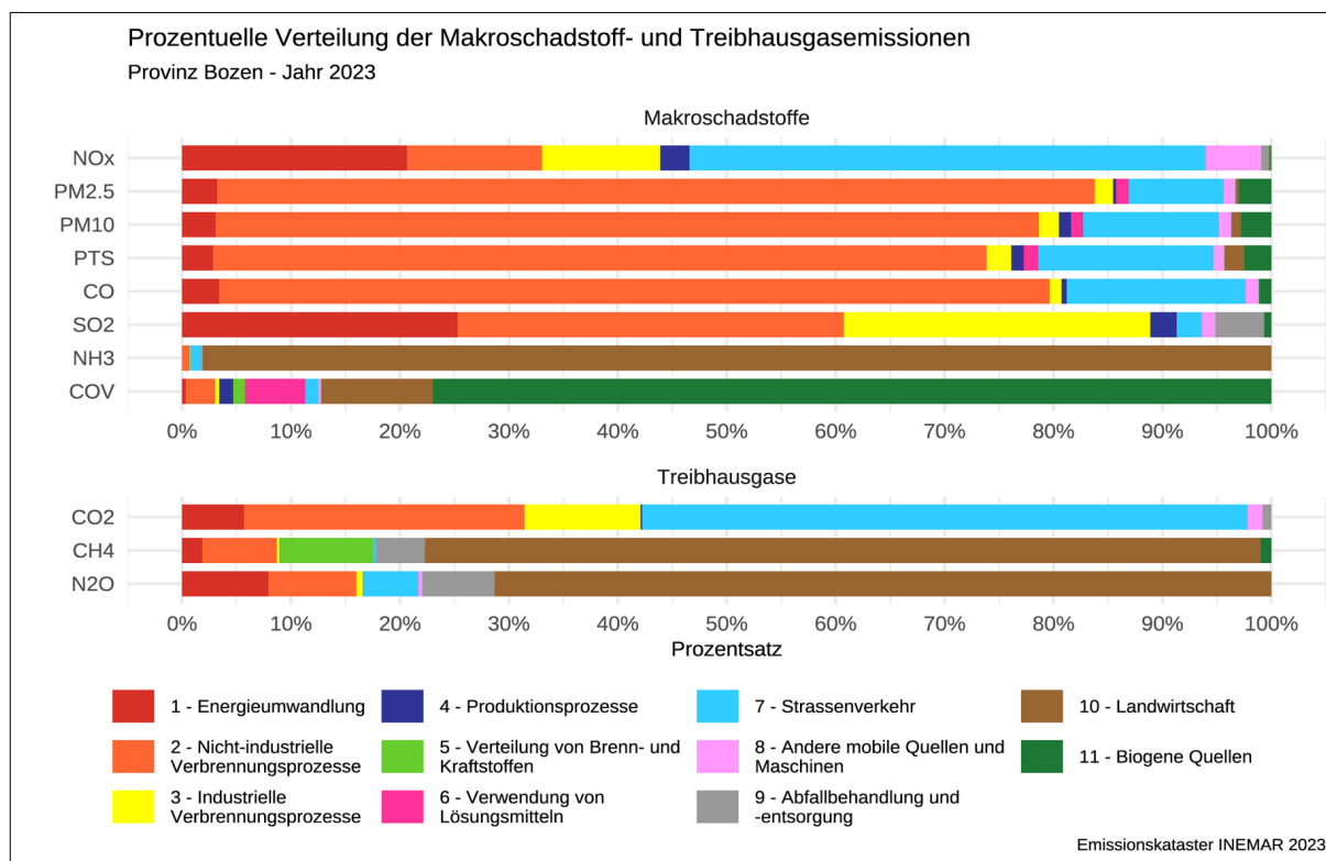
Abbildung 1: Prozentuelle Verteilung der Makroschadstoff- und klimarelevanten Gasemissionen im Jahre 2023 1
