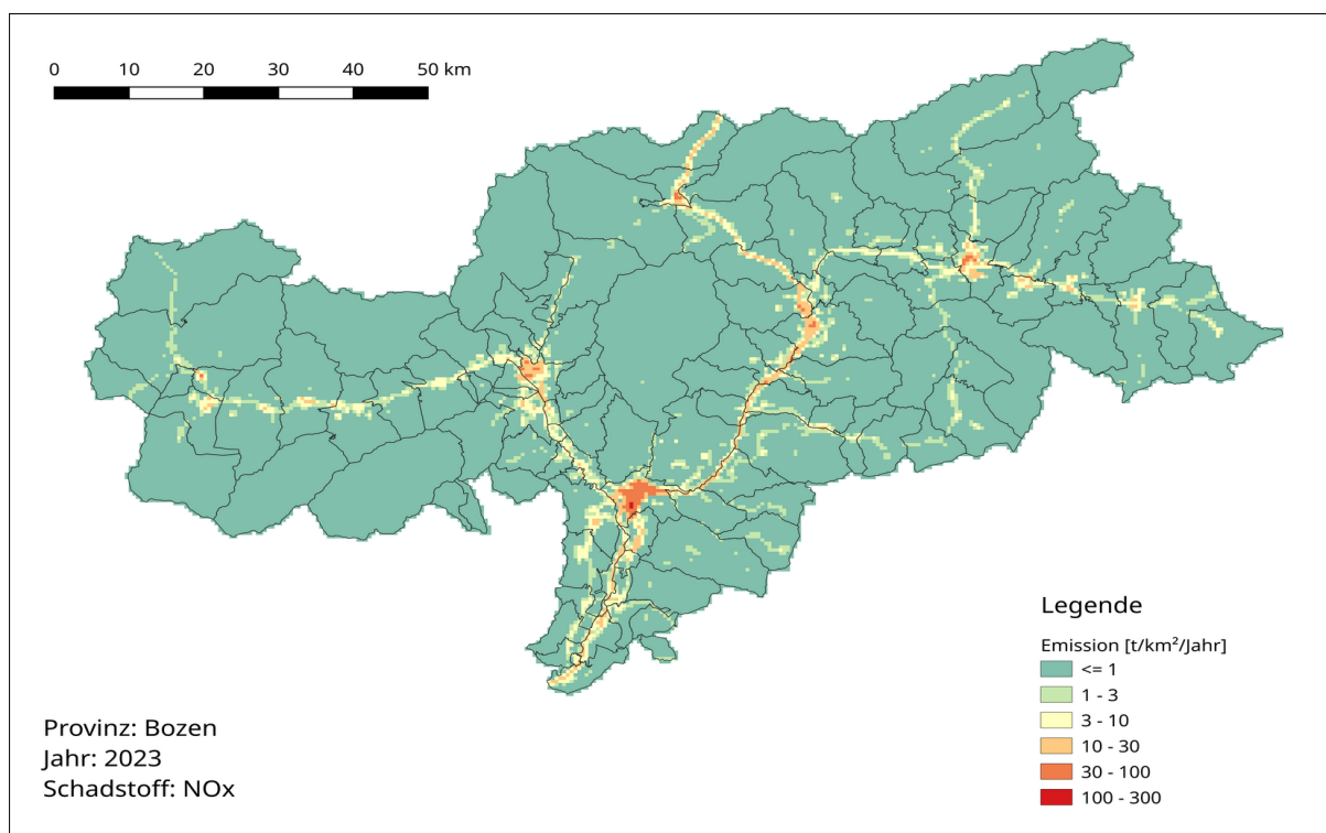
Abbildung 6: Räumliche Verteilung der \text{NO}_x -Emissionen im Jahre 2023
