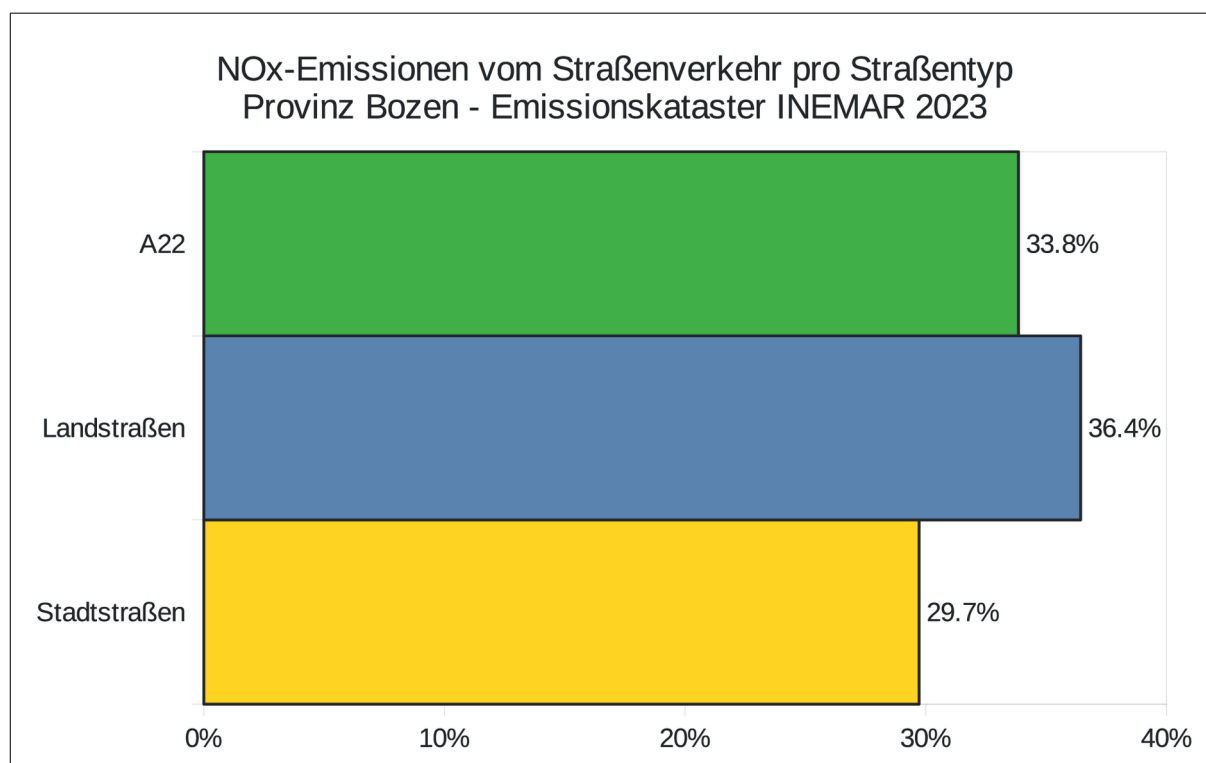
Abbildung 5: Anteil unterschiedlicher Straßentypen an der Emission von NO x (Jahr 2023)
