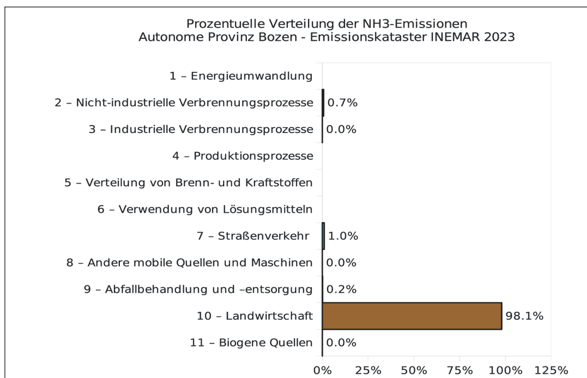
Abbildung 10: Prozentuelle Verteilung der NH 3 -Emissionen (Jahr 2023)
