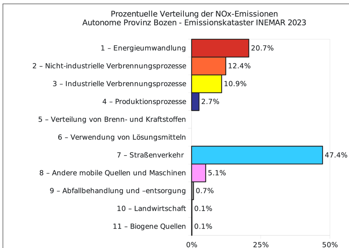
Abbildung 3: Prozentuelle Verteilung der NO x -Emissionen (Jahr 2023)
