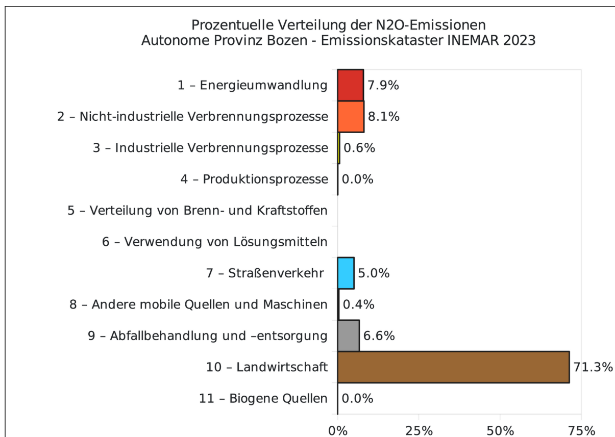
Abbildung 17: Prozentuelle Verteilung der N 2 O-Emissionen (Jahr 2023)
