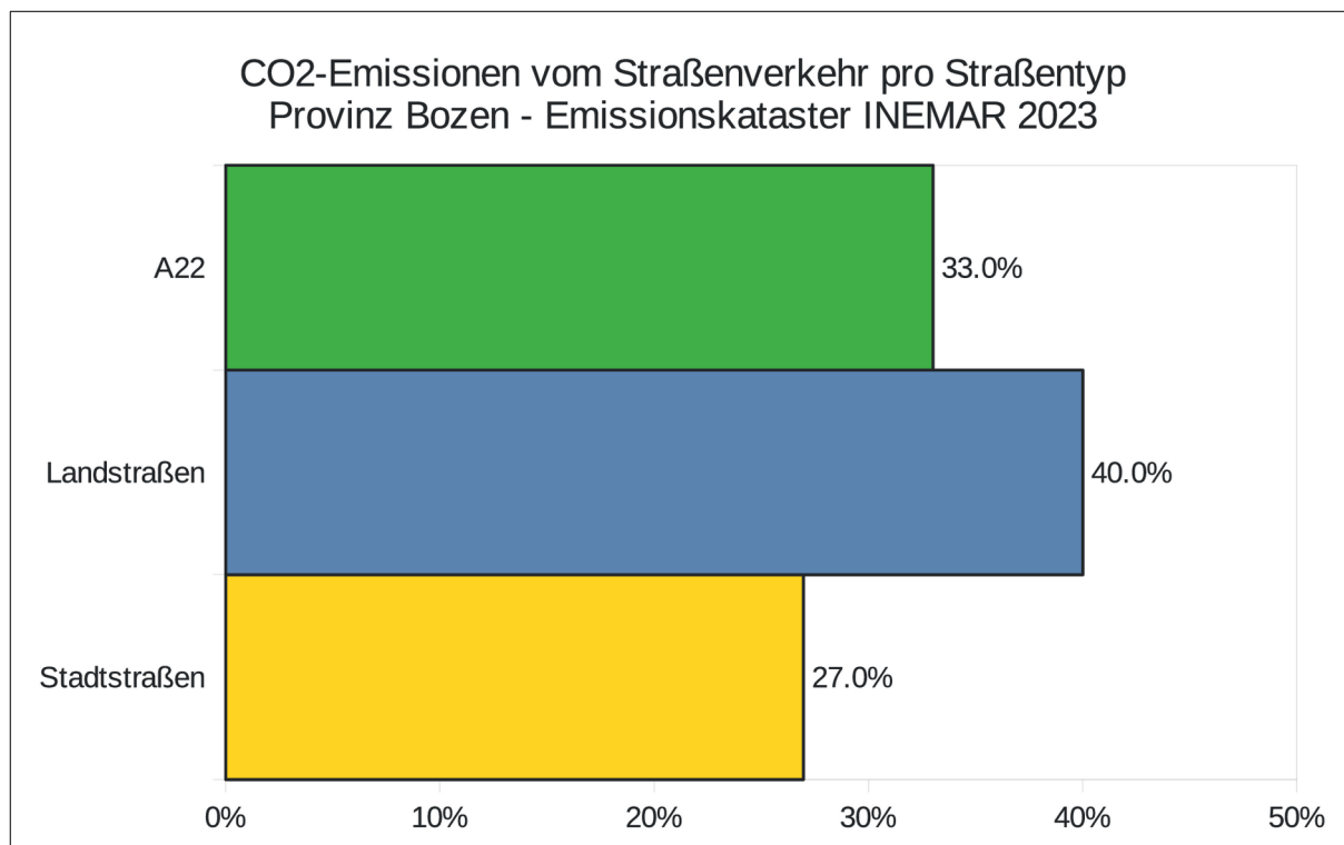
Abbildung 15: Anteil der CO 2 -Emissionen vom Verkehr (2023) unterschiedlicher Straßentypen
