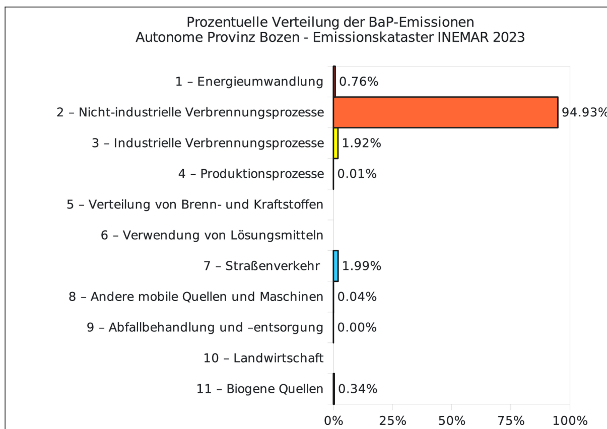
Abbildung 12: Prozentuelle Verteilung der B(a)P-Emissionen (Jahr 2023)
