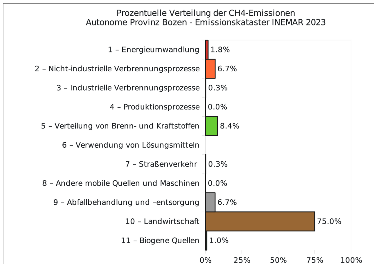
Abbildung 16: Prozentuelle Verteilung der CH 4 -Emissionen (Jahr 2023)
