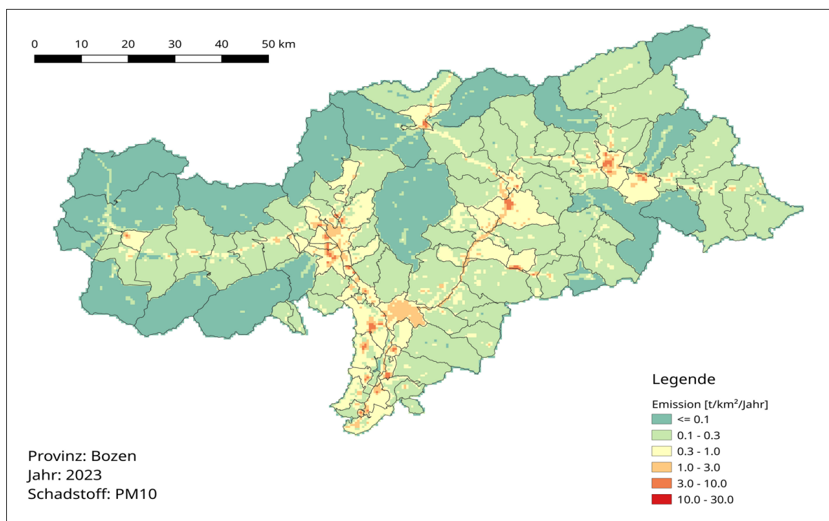
Abbildung 8: Räumliche Verteilung der PM10-Emissionen im Jahre 2023
