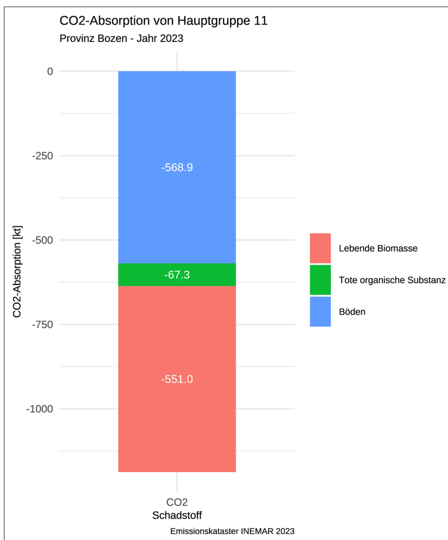
Abbildung 22: CO 2 -Absorption von Hauptgruppe 11
