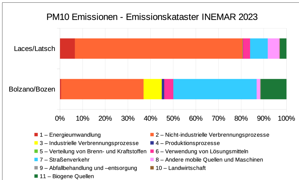
Abbildung 9: Vergleich der PM10-Emissionen nach Typ der Emissionsquelle in den Gemeinden Latsch und Bozen (2023)
