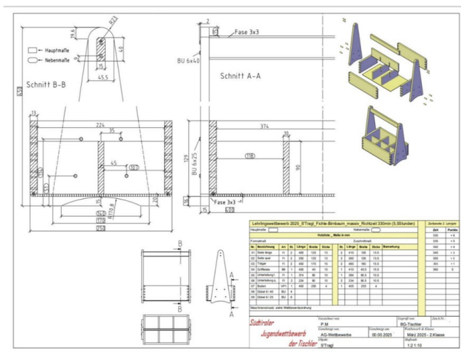
Fertigungsplan für die 2. Klasse: „S'Tragl“ (Flaschenträger)
