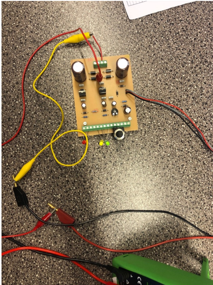
Netzteil und der Arbeitsplatz im Labor
