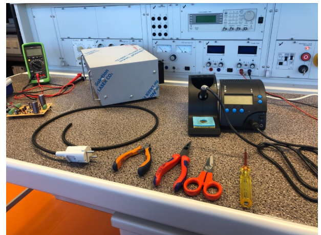
Netzteil und der Arbeitsplatz im Labor
