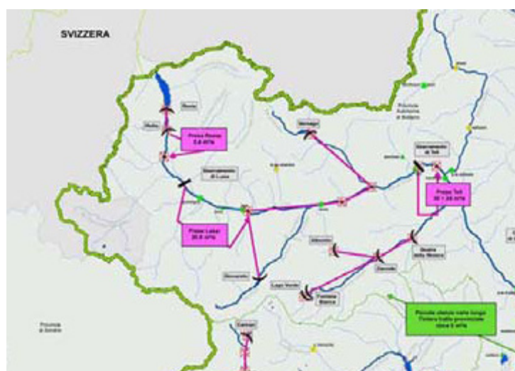
Figura 87d: schema idraulico derivazioni ed adduzioni idroelettriche Val Venosta (fonte: Ripartizione Agricoltura)
