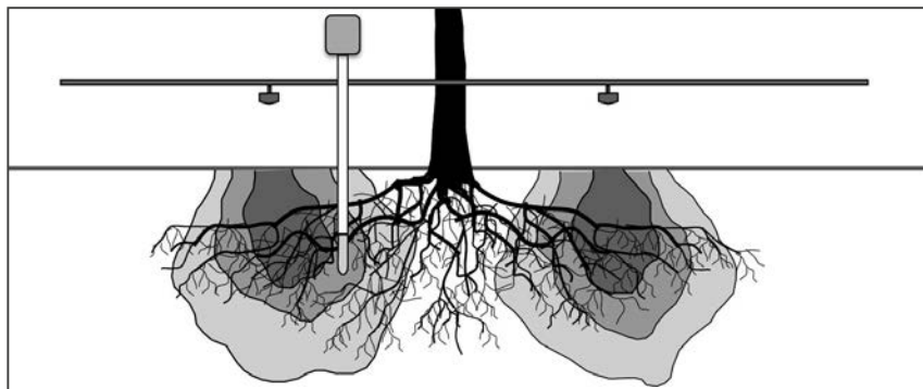
Abb. 2: Installierte Bodenfeuchtesensoren im Obstbau zur Messung der Saugspannung im Boden
