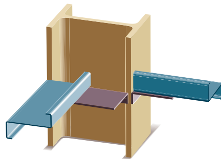
Abbildung c - Wandriegel zwischen Sparren
