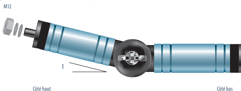
Regelbarer Abstandshalter mit Nylonkappe
