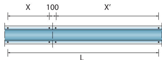
Verbindungsstück Innenfeld (SLE)
