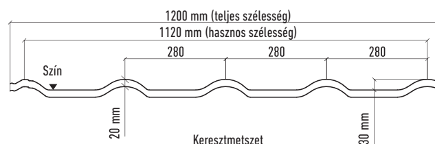
Keresztmetszet
