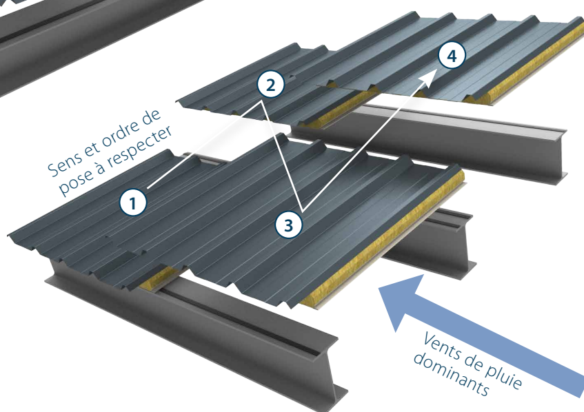
Figure 33 : Sens de pose pour panneau type «gauche»
