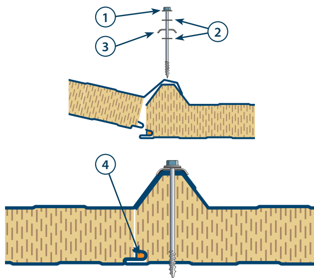
Figure 31 : Rive emboîtante et emboîtée
