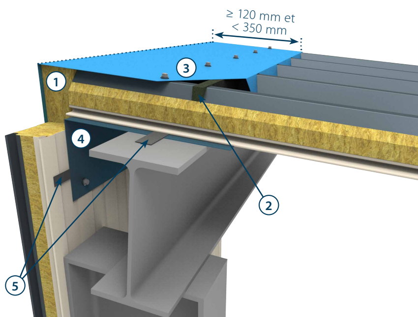
Figure 44 : Faîtière simple
