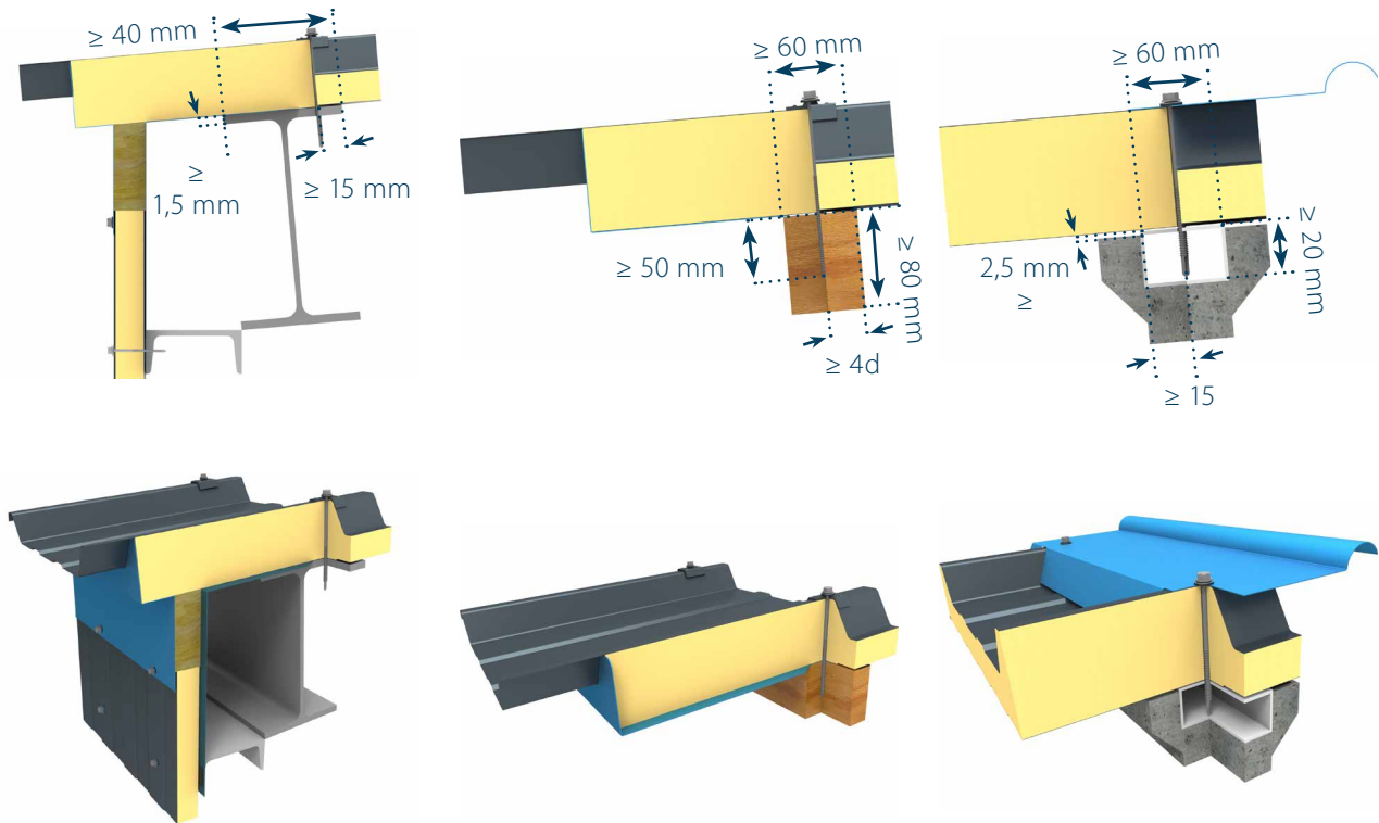
Figure 7 : Appuis d'extrémité
