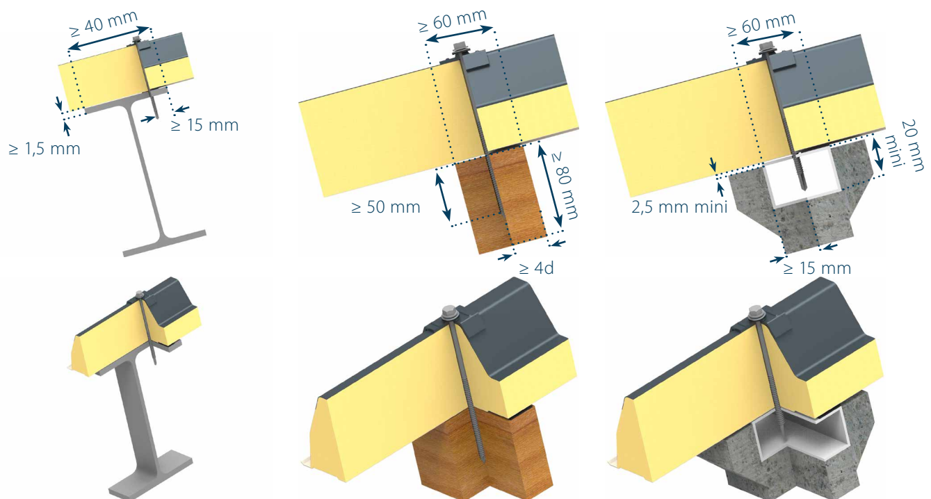
Figure 6 : Appuis intermédiaire
