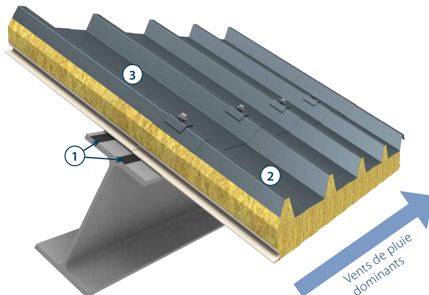
Figure 38 : Joints sur appuis au droit d'un recouvrement transversal sans complément d'étanchéité (CE) - locaux à faible ou moyenne hygrométrie
