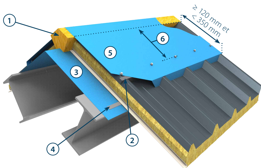
Figure 43 : Faîtière double
