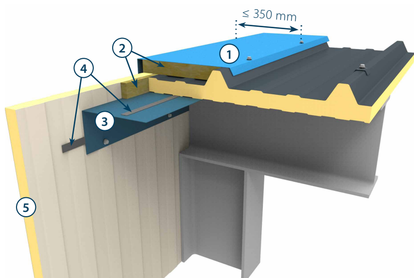
Figure 26 : Rive contre pignon
