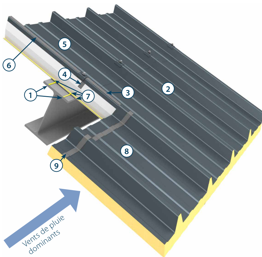
Figure 12 : Joints sur appuis au droit d'un recouvrement transversal de panneaux avec complément d'étanchéité transversal et longitudinal - locaux climatisés
