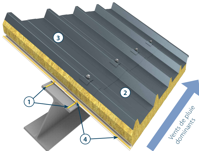
Figure 40 : Joints sur appuis au droit d'un recouvrement transversal sans complément d'étanchéité (CE) - locaux climatisés
