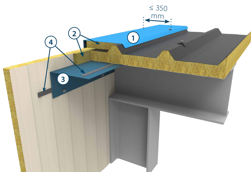
Figure 53 : Rive contre pignon
