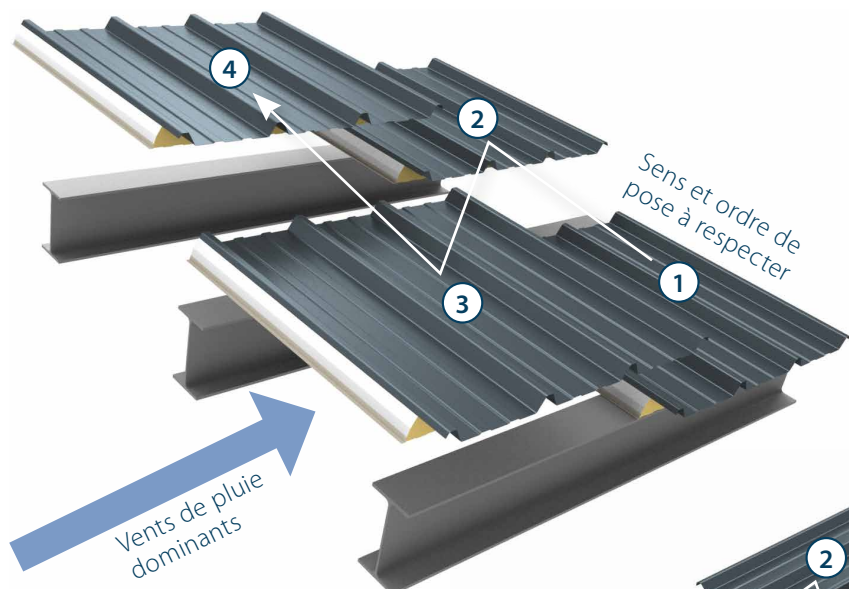
Figure 3 : Sens de pose pour panneau type «droit»
