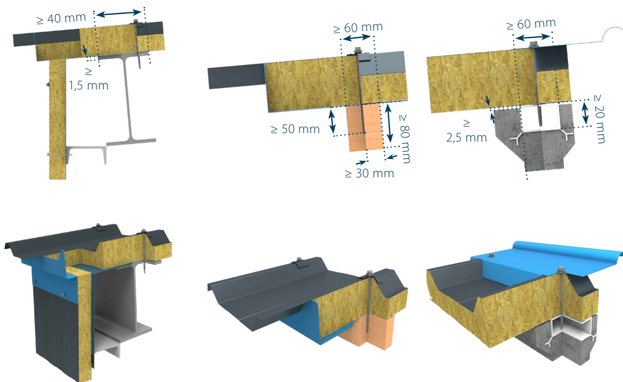
Figure 36 : Appui extrémité
