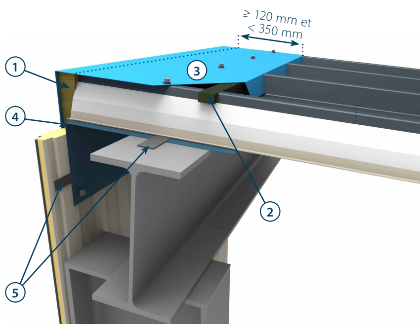
Figure 17 : Faîtière simple sans dépassement de toiture
