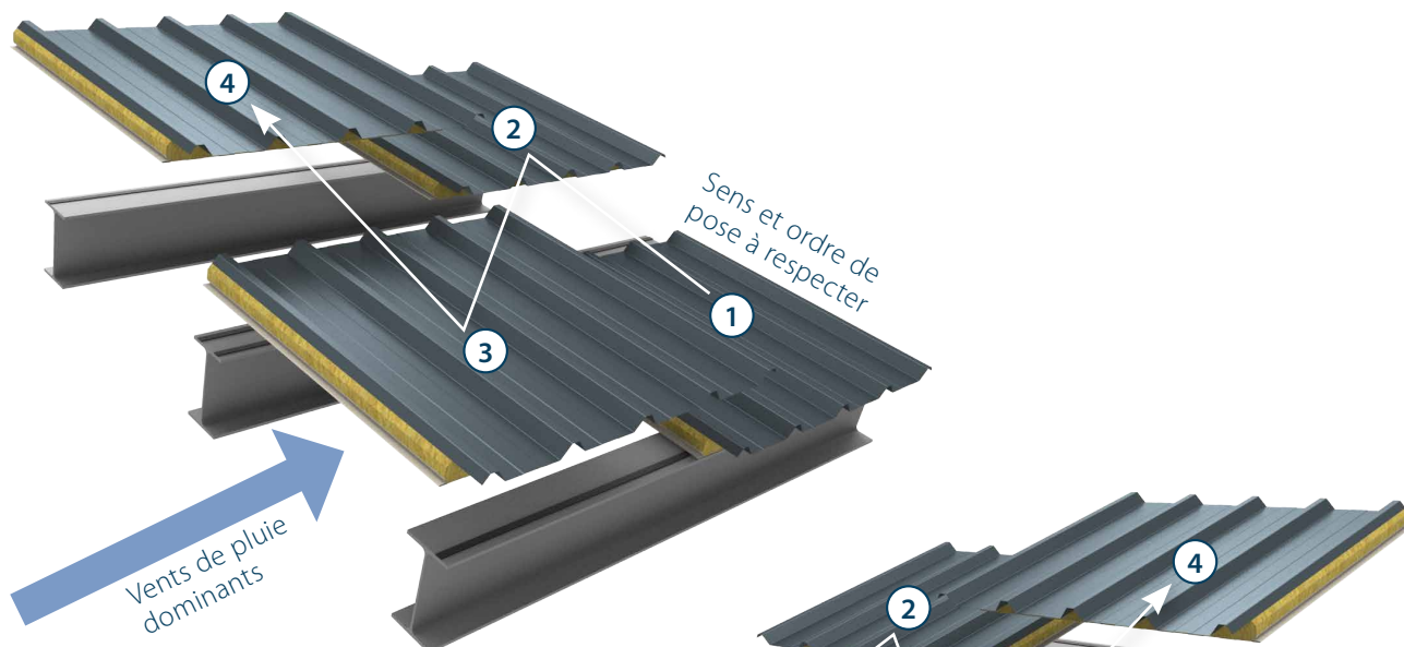
Figure 32 : Sens de pose pour panneau type «droit»
