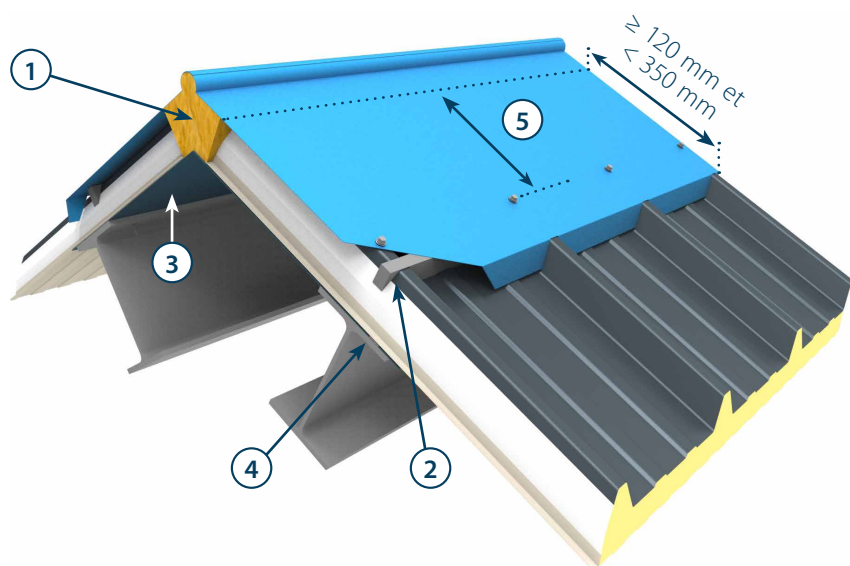
Figure 15 : Faîtage articulé avec demi-faitière à boudin
