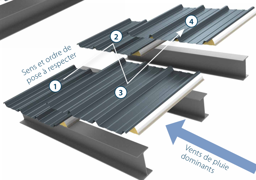
Figure 4 : Sens de pose pour panneau type «gauche»
