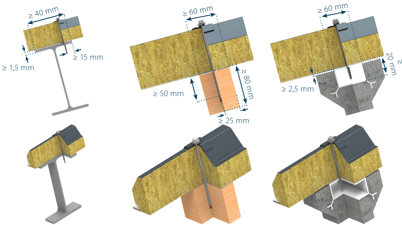
Figure 35 : Appui intermédiaire
