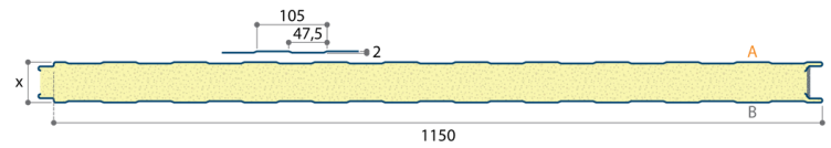
Nieuwe geometrie van de Eurobox
