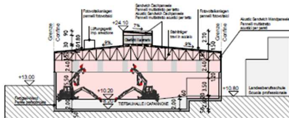
SNITT B-B SEZIONE B-B
