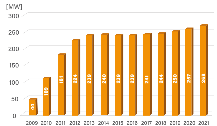
Abbildung 16 - Gesamtleistung der installierten PV-Anlagen - Quelle: GSE
