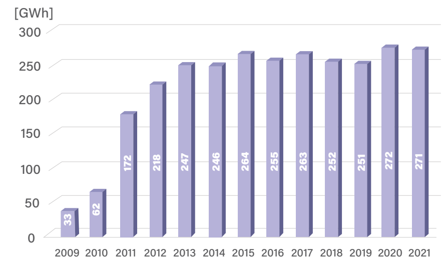
Abbildung 17 - Stromproduktion aus Photovoltaikanlagen - Quelle: GSE
