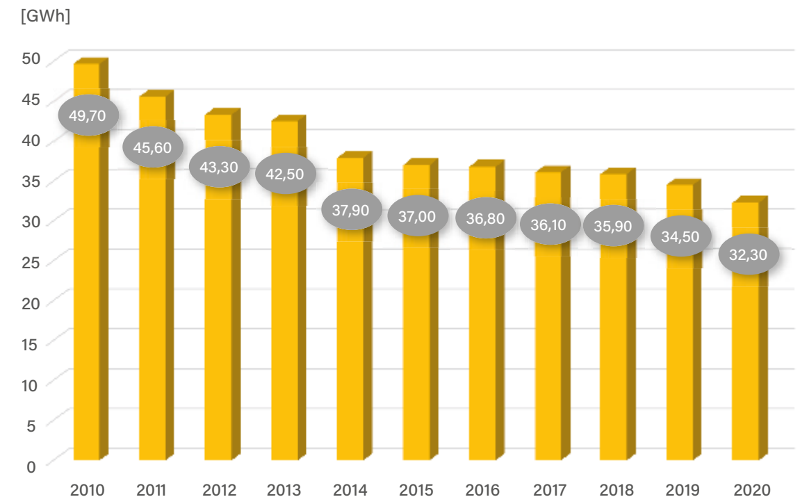
Abbildung 23 - Stromverbrauch für die öffentliche Beleuchtung in Südtirol
