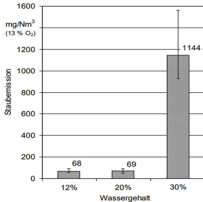
Gesamtstaubemission
