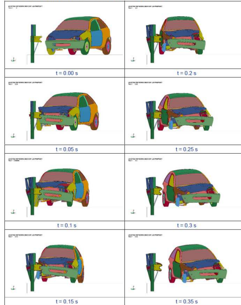
7.1.3 IMMAGINI DELLA SIMULAZIONE TB11 DI CALIBRAZIONE
