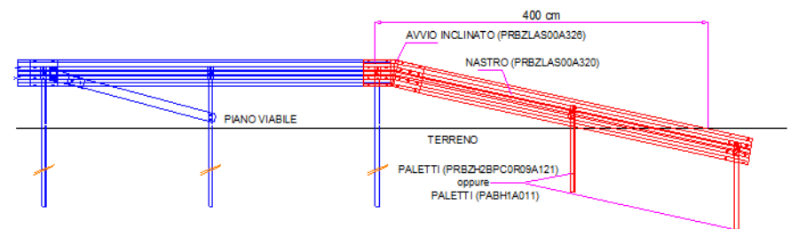
Gruppo terminale installato durante crash test PAB N2 T2 e T4
