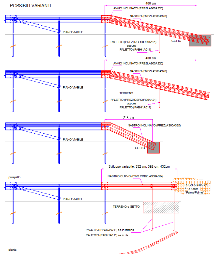
Gruppo terminale installato durante crash test PAB N2 T2 e T4
