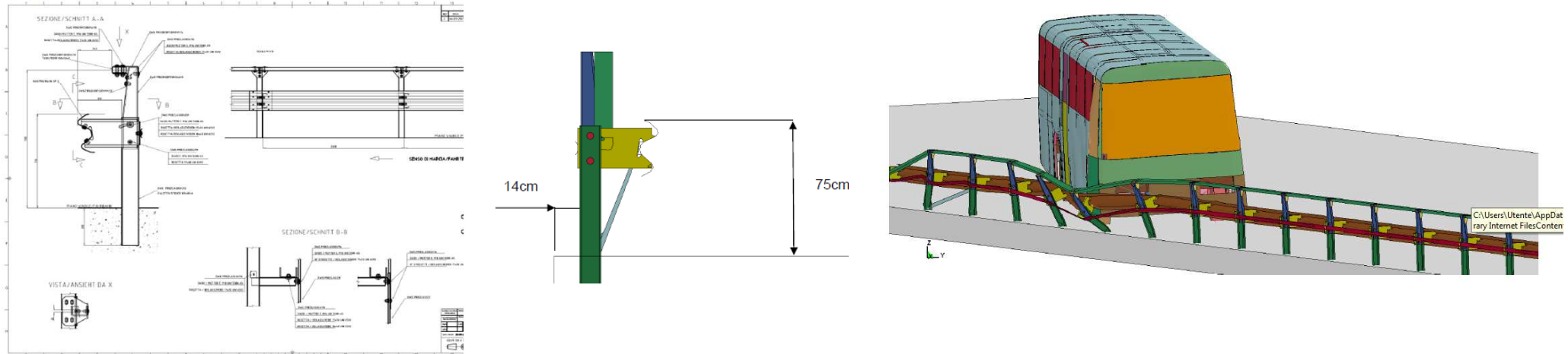
7.1.7 IMMAGINI DELLA SIMULAZIONE TB51 DI CALIBRAZIONE
