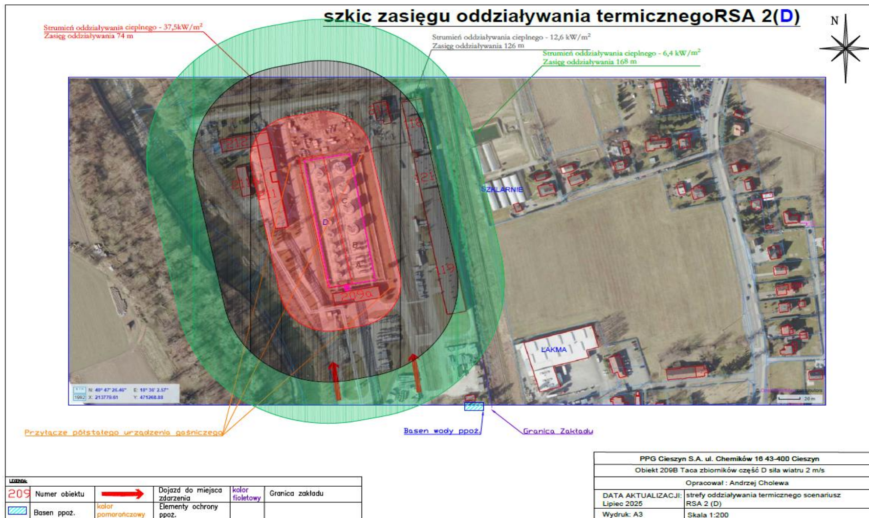
Rysunek 6. RSA 2D.
