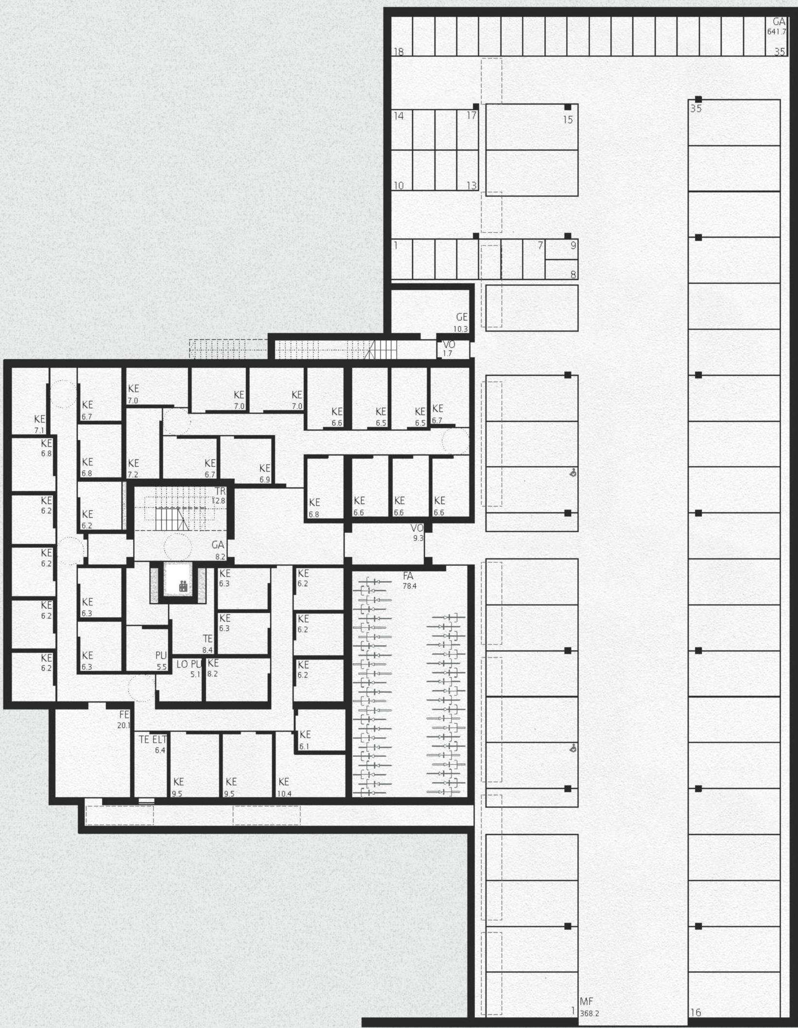
UNTERGESCHOSS 1|200
