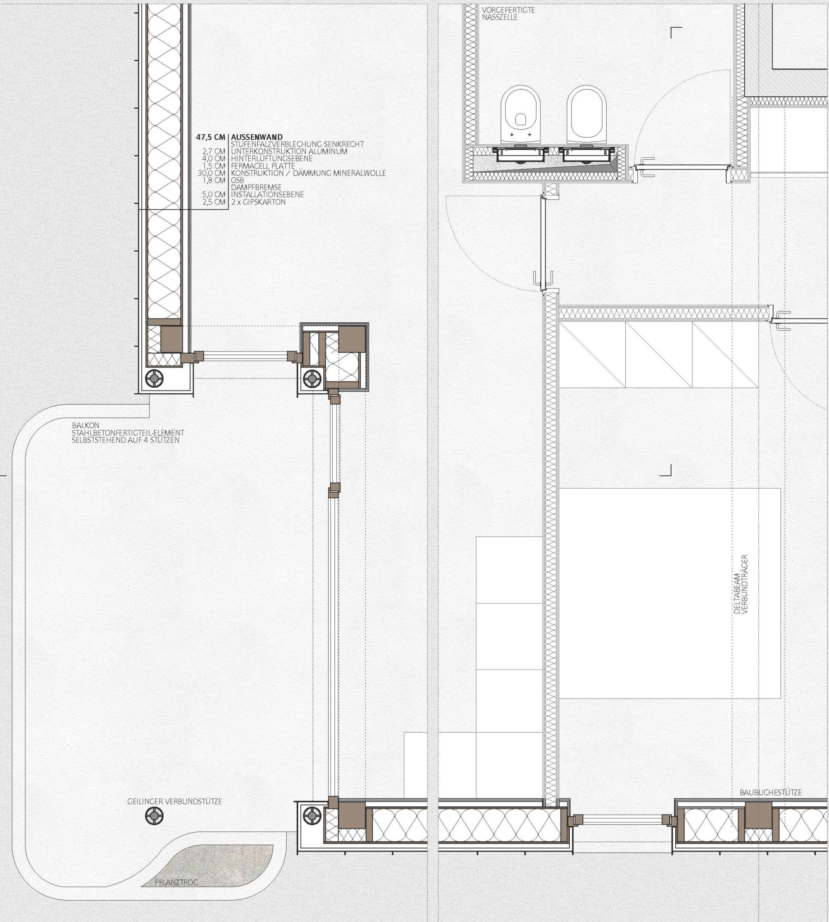
DETAILSNITT - GRUNDRISS 1|20
