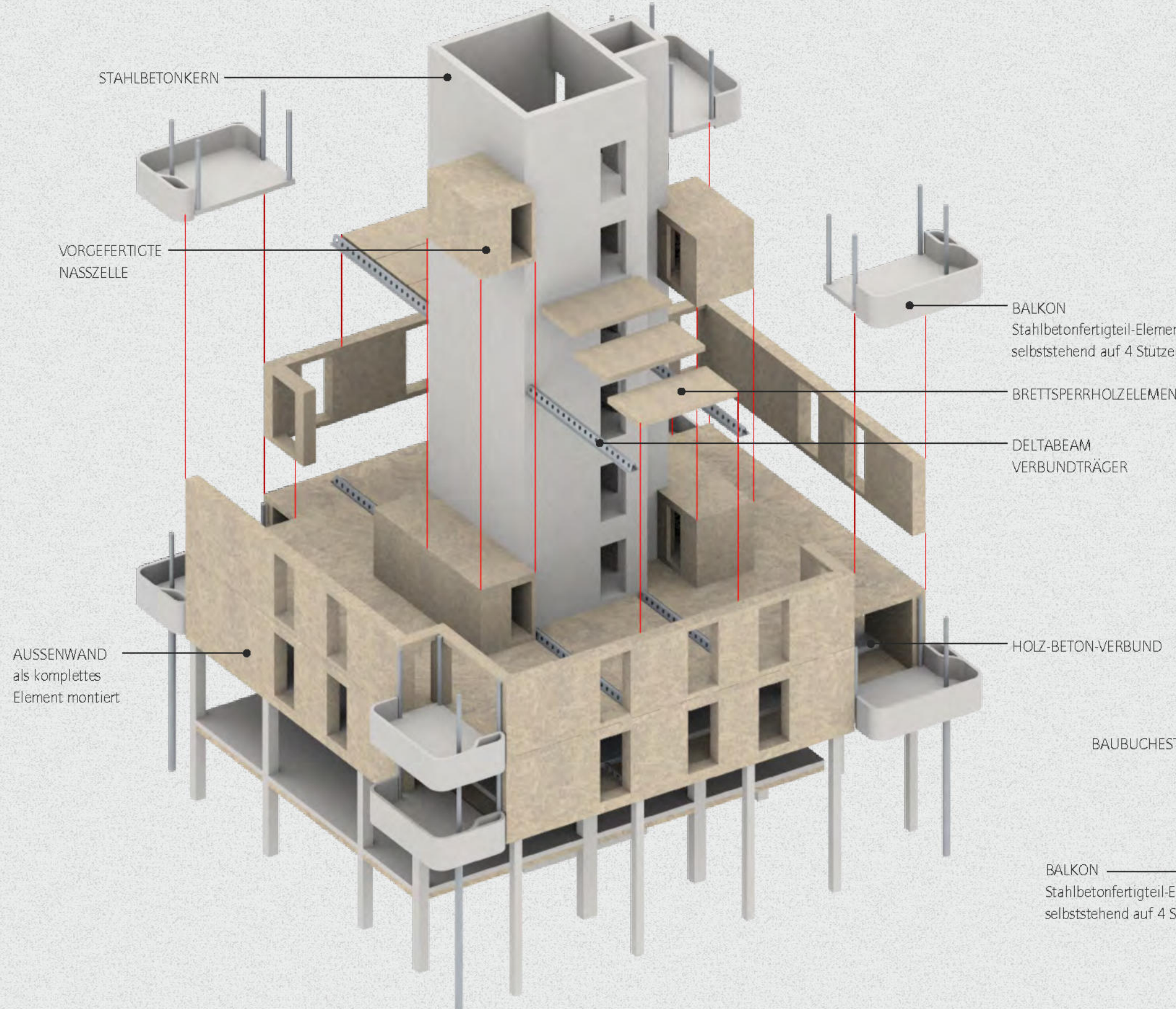
MONTAGEKONZEPT
