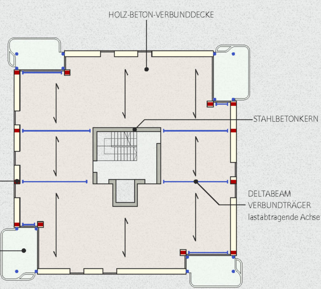
TRAGWERKS-KONZEPT 1|200
