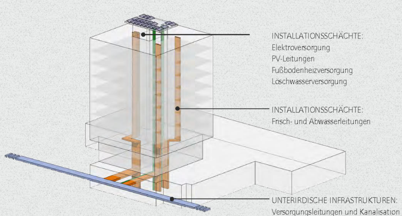
HLSE - KONZEPT
