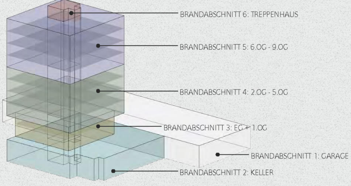
BRANDSCHUTZ-KONZEPT
