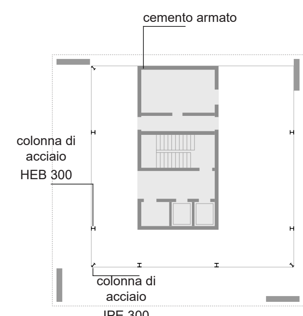
CONCETTO STRUTTURALE
