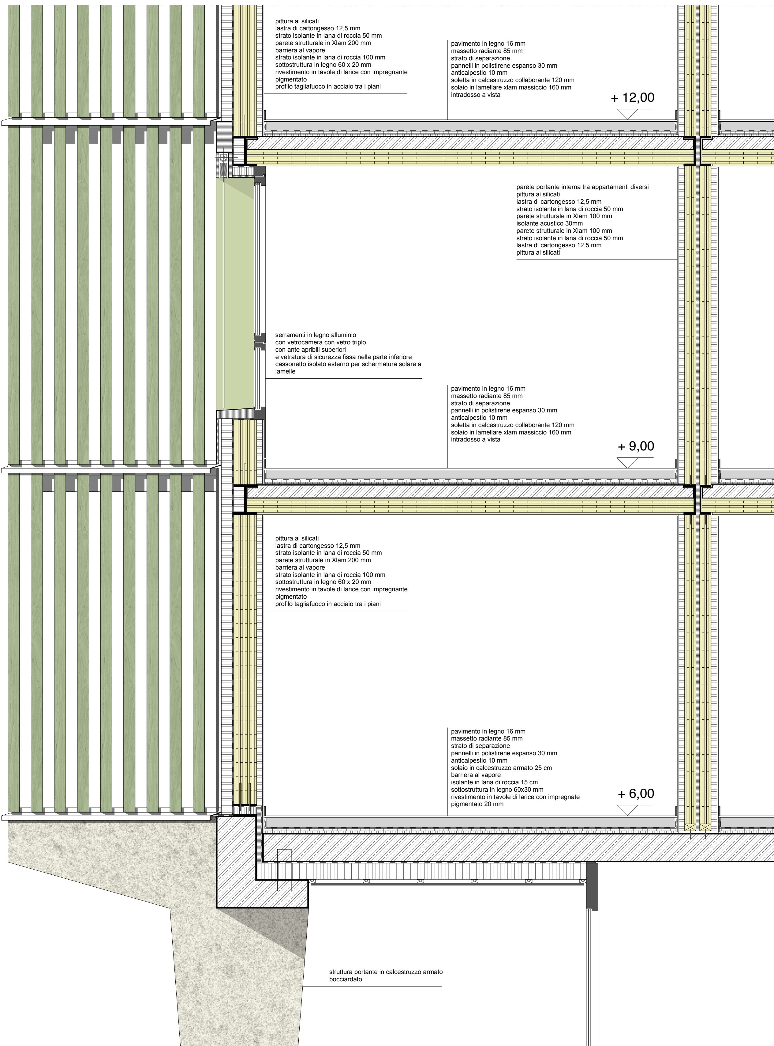
SEZIONE DI FACCIA CON STRATIGRAFIE E DETTAGLI DEI NODI 1:20
