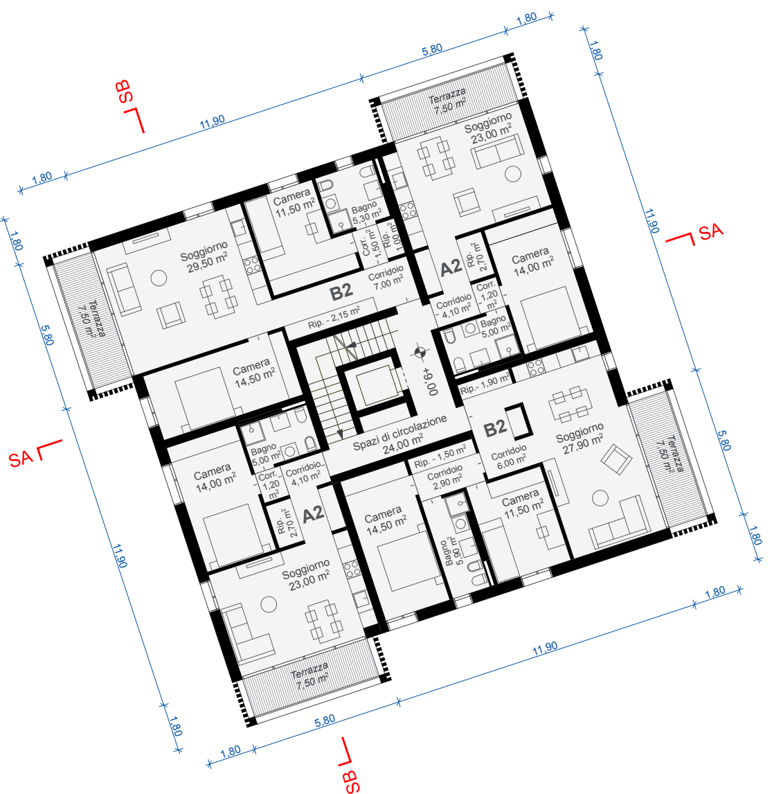
3°, 5°, 7° E 9° PIANO 1:200
