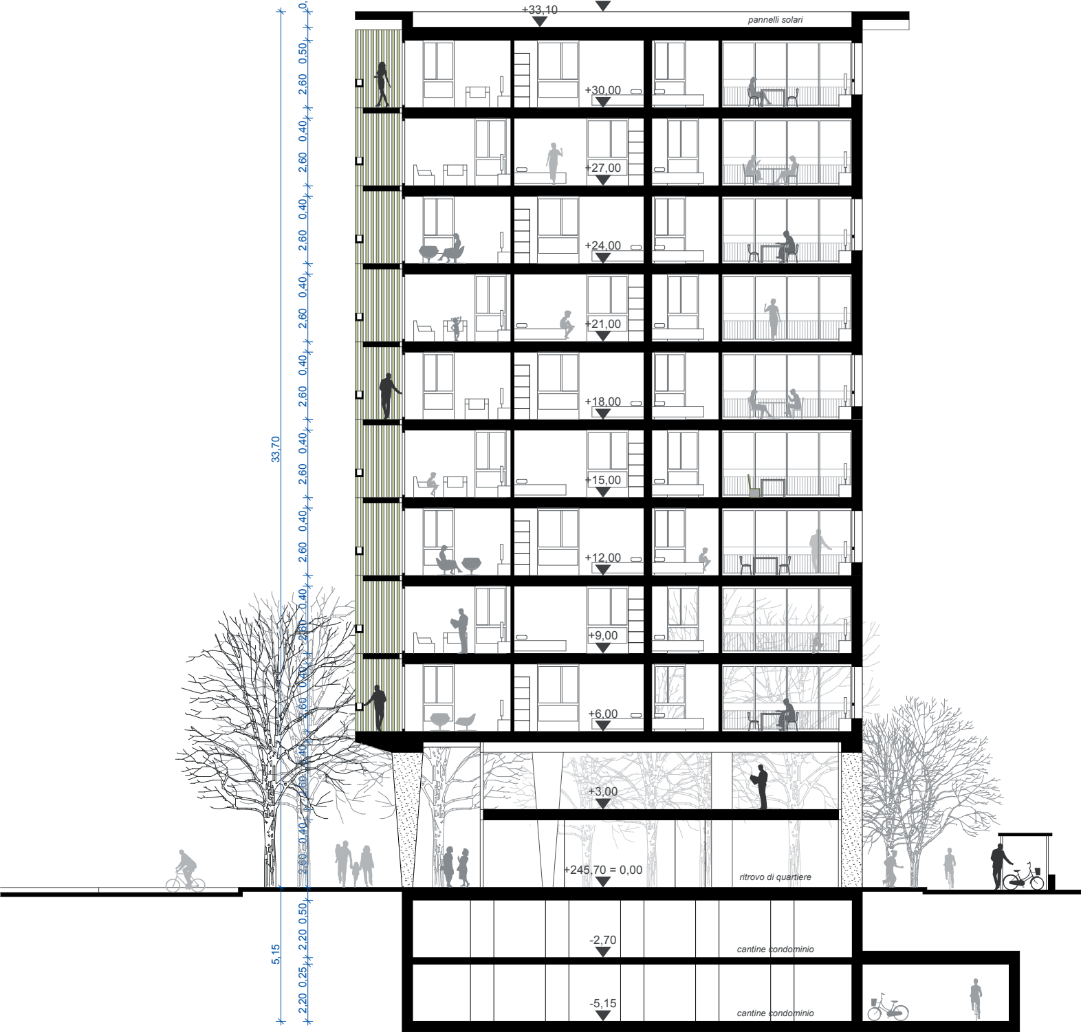
SEZIONE SB 1:200
