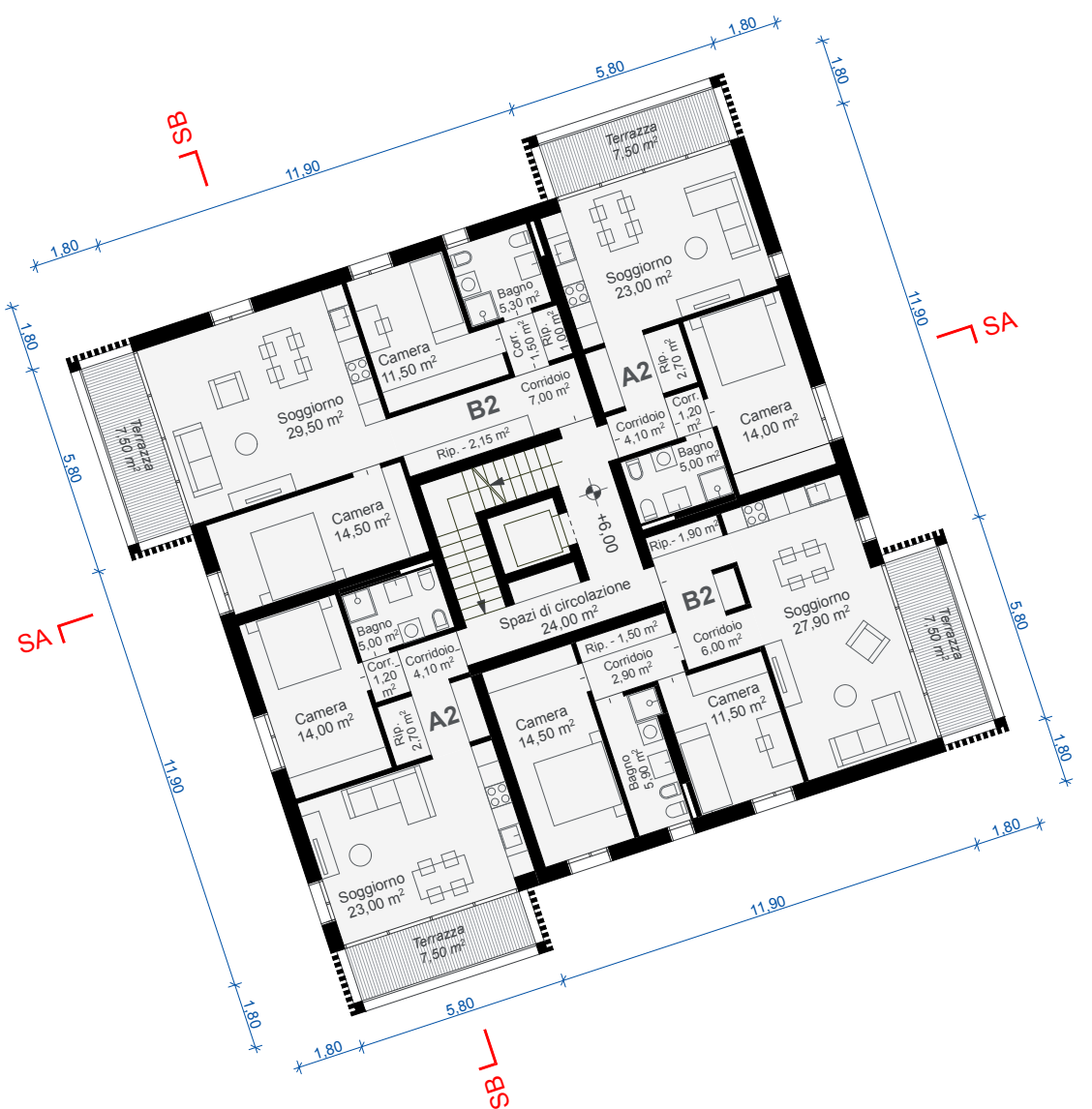
2° E 8° PIANO 1:200
