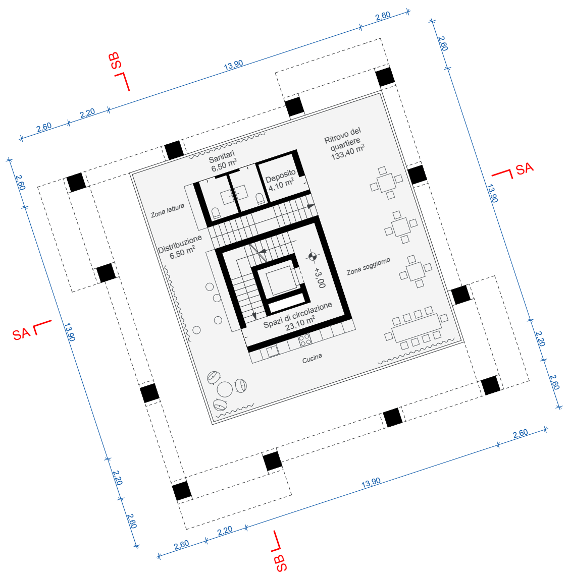
1° PIANO 1:200
