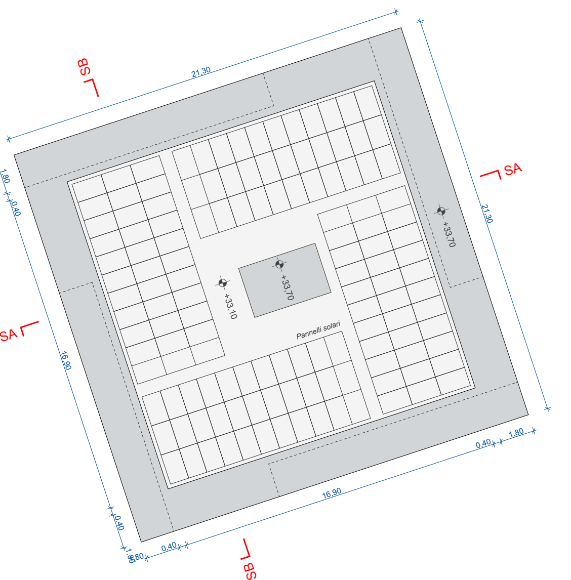
PIANO DELLA COPERTURA 1:200
