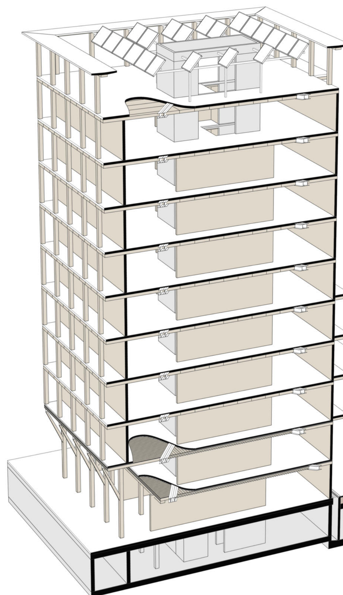
SCHEMA STRUTTURALE - ASSONOMETRICO
