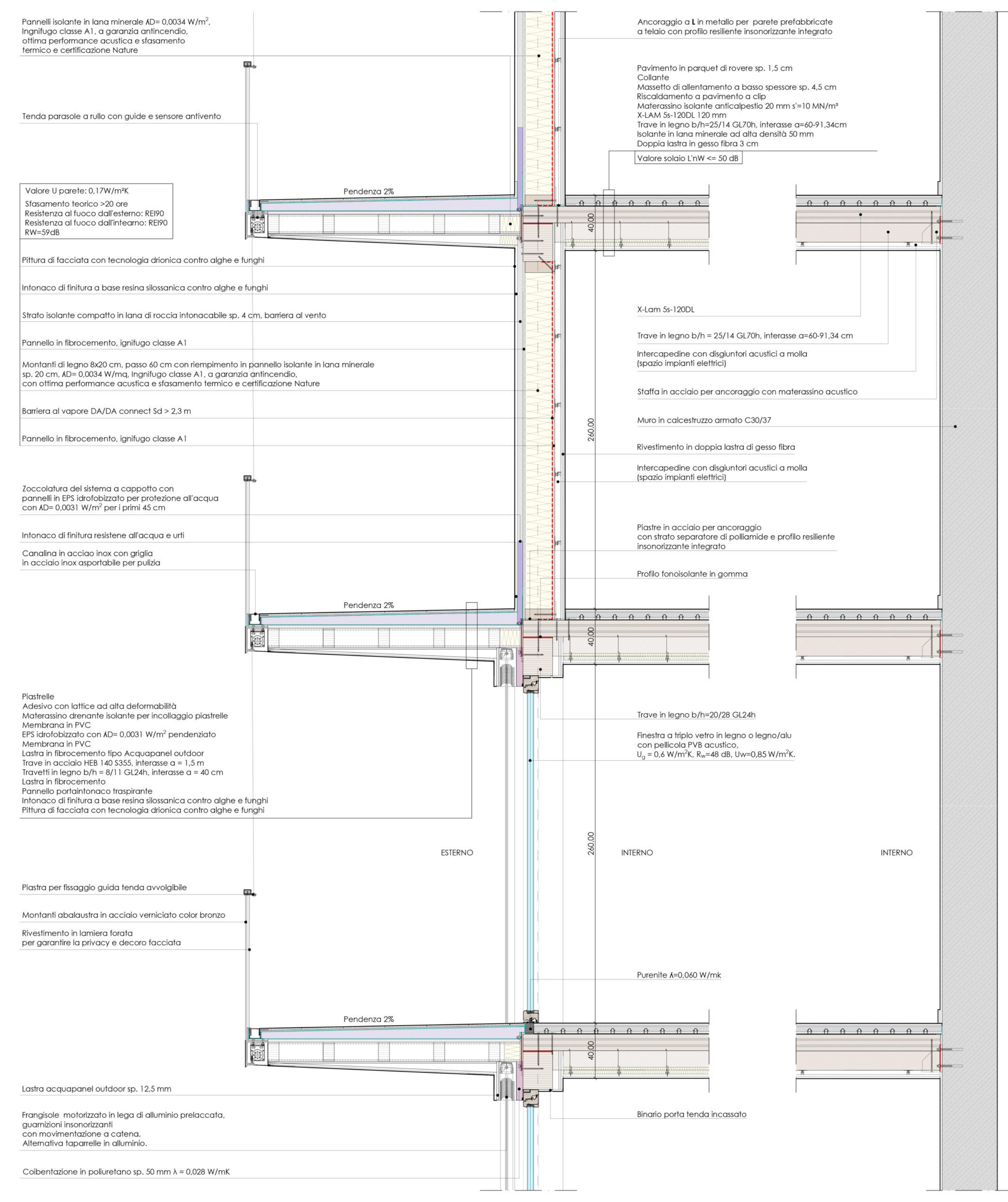
SEZIONE FACCIAIA
