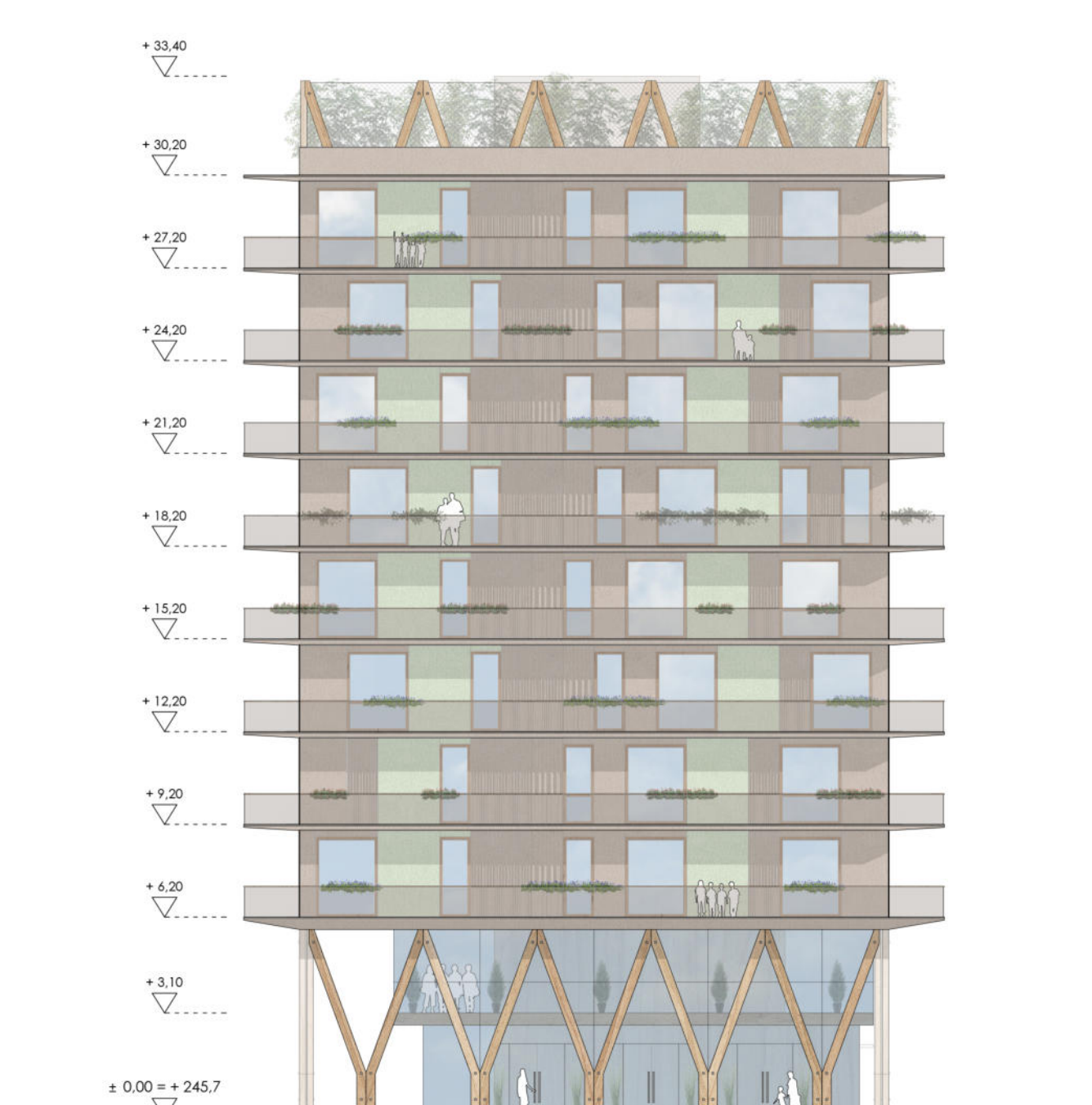
PROSPETTO EEN
