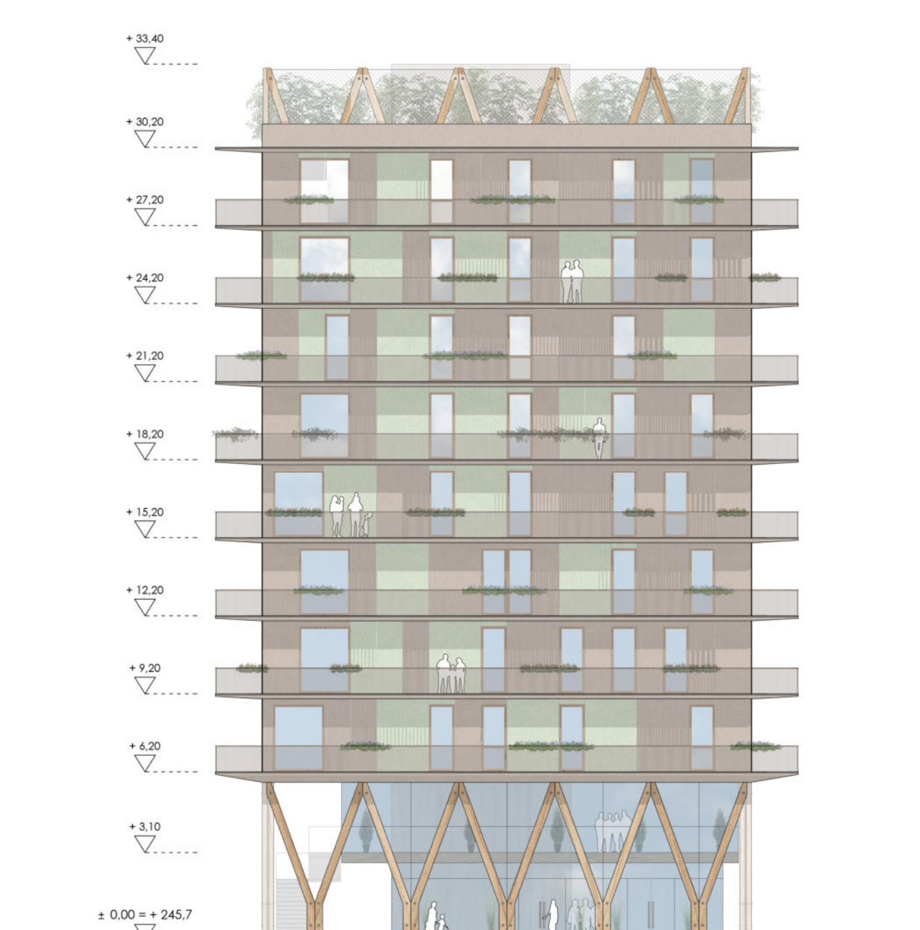
PROSPETTO SSE
