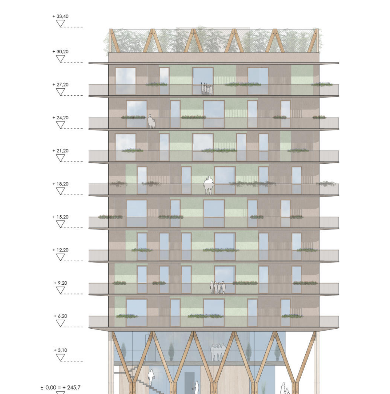
PROSPETTO OOS
