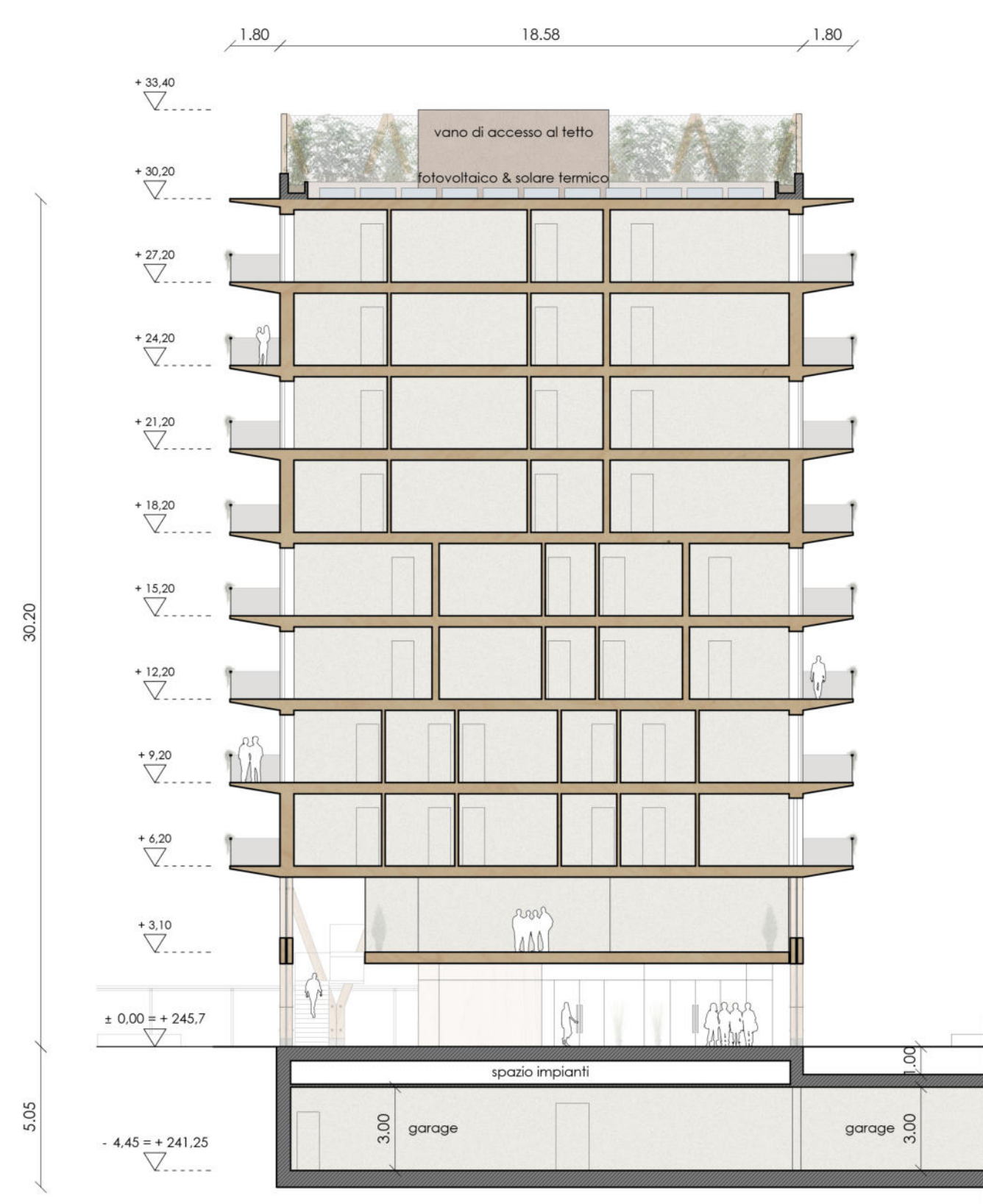
SEZIONE A-A
