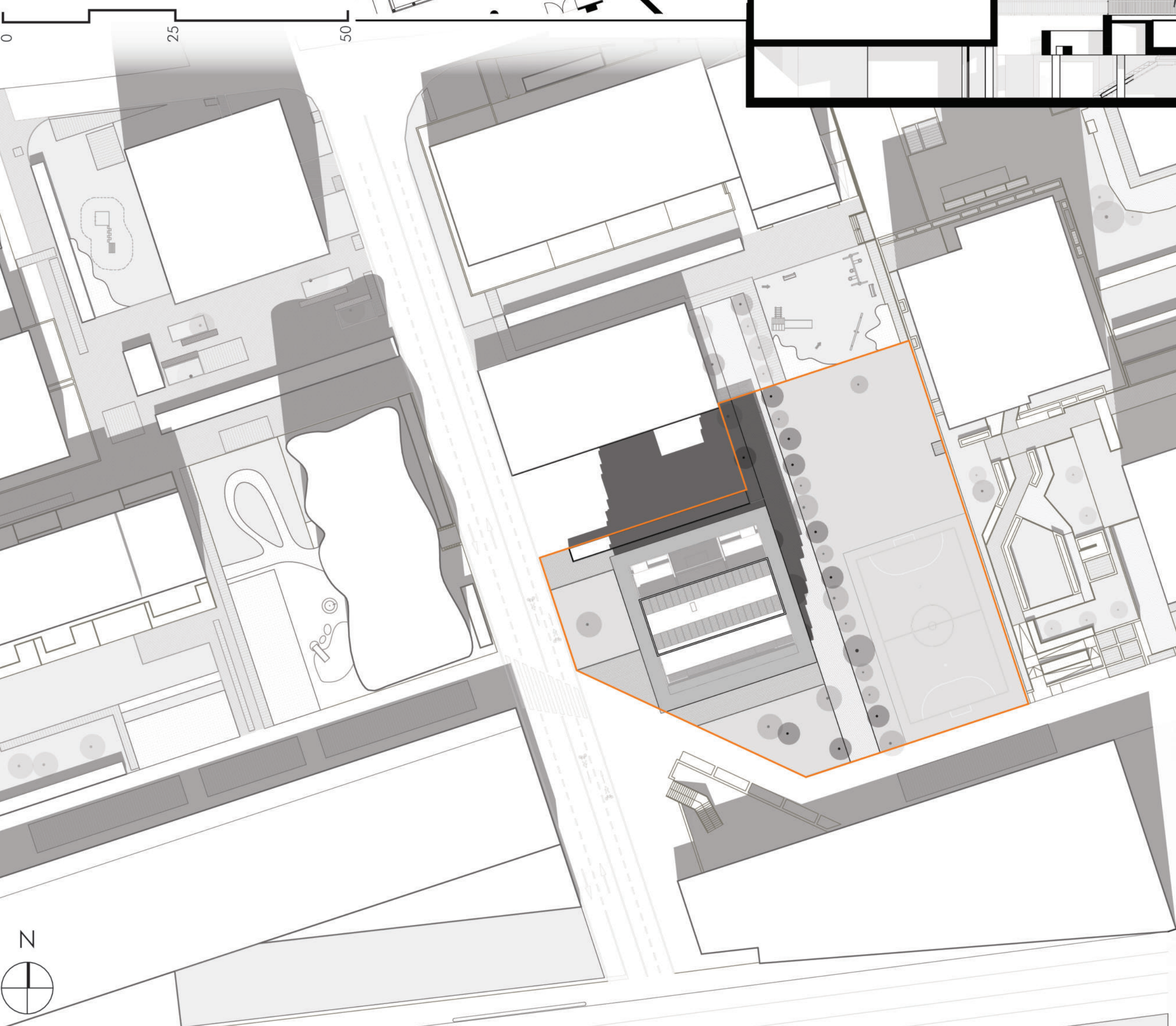
Planimetria generale
