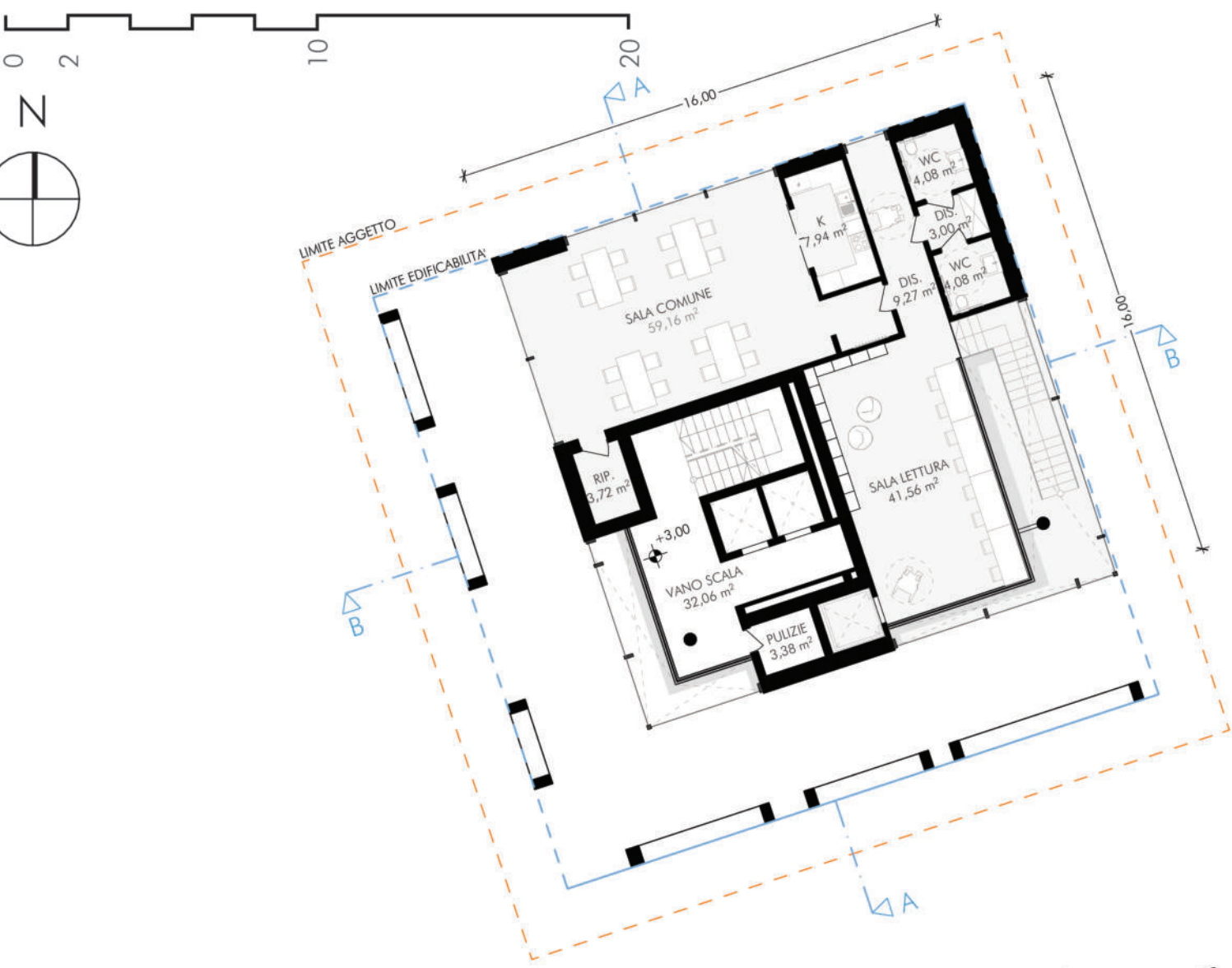
Piano 1°
