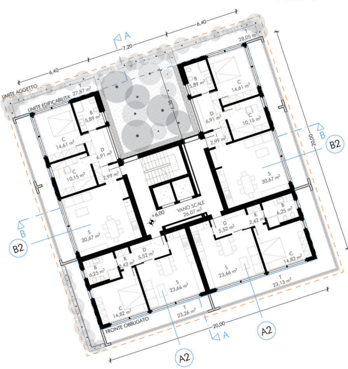
Piano 2°
