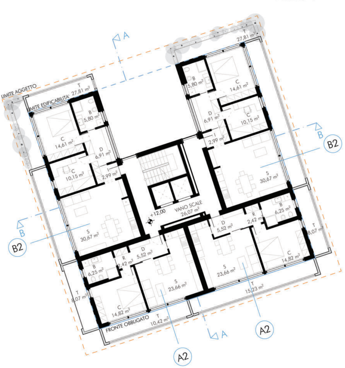
Piano 4°
