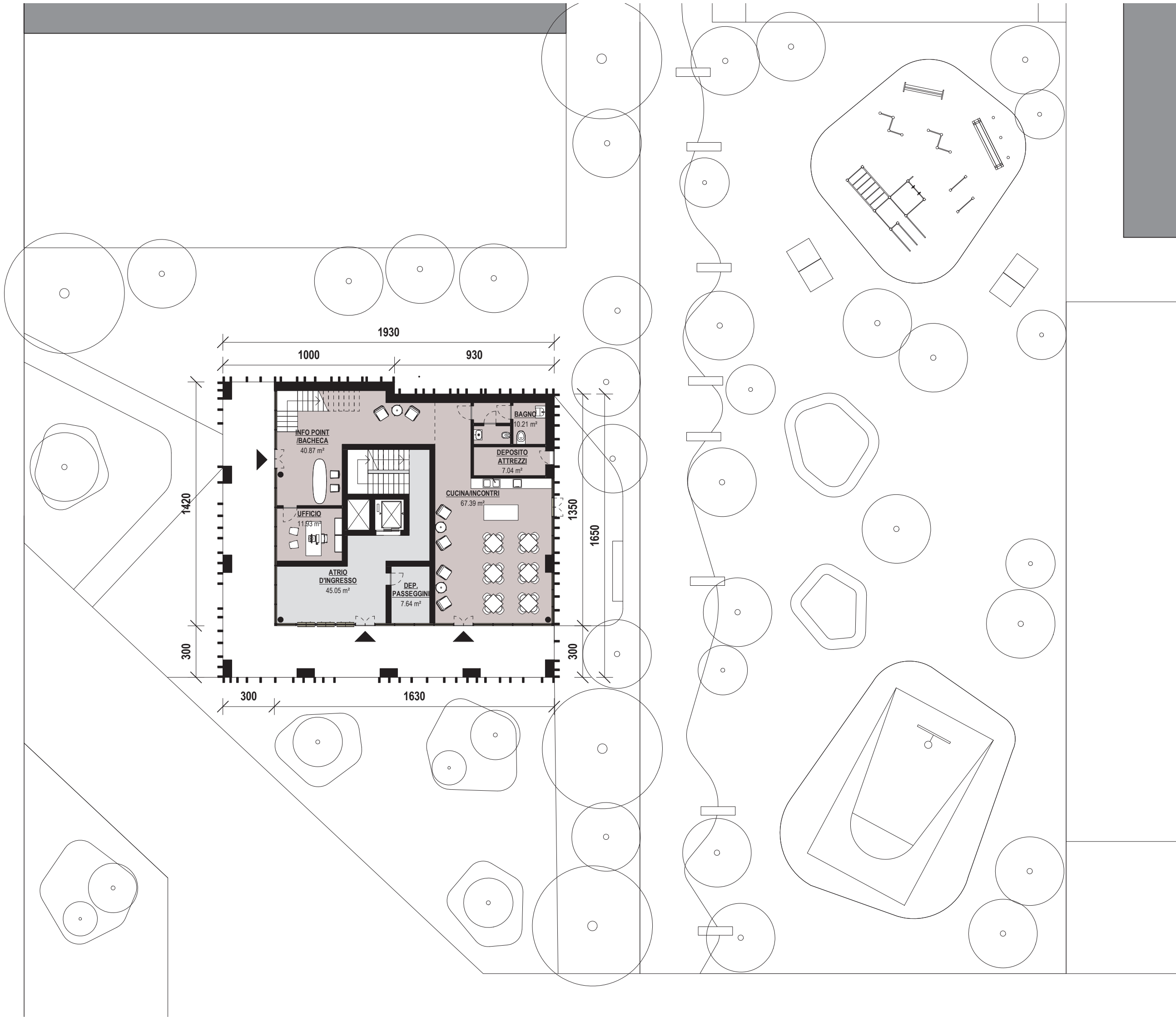
PIANO TERRA SCALA 1:200
