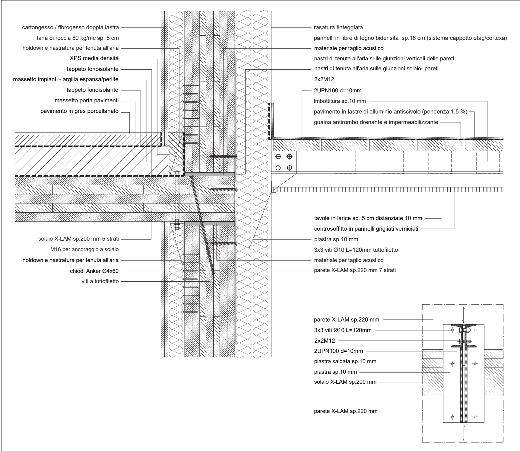
nodo solaio parete esterna in X-LAM
