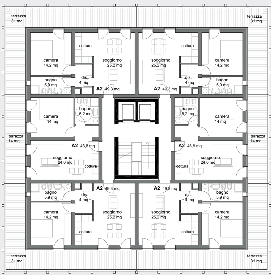
piano secondo - terzo
