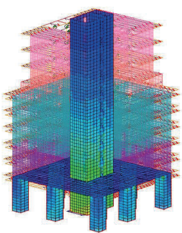
verifica porzione di struttura in cemento armato
