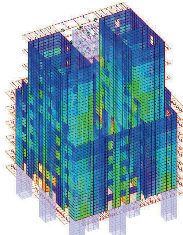
verifica porzione di struttura in xlam (prestressione)
