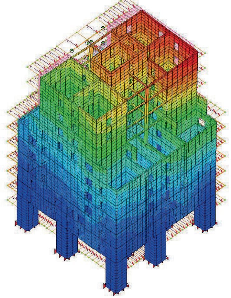
massima deformazione sotto sisma
