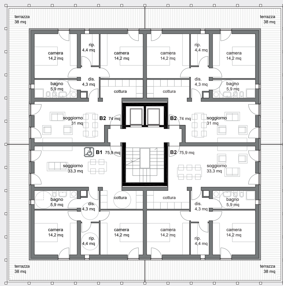
piano quarto - quinto - sesto
