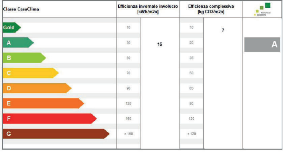
classificazione preliminare di calcolo CasaClima
