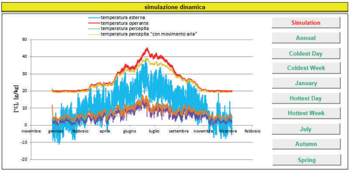
calcolo dinamico delle temperature dell'edificio
