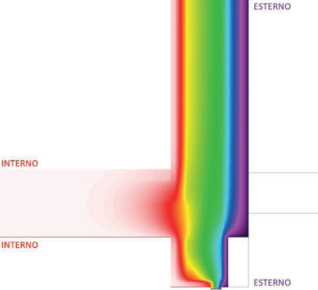
calcolo agli elementi finiti del ponte termico del nodo parete-terrazza-finestra
