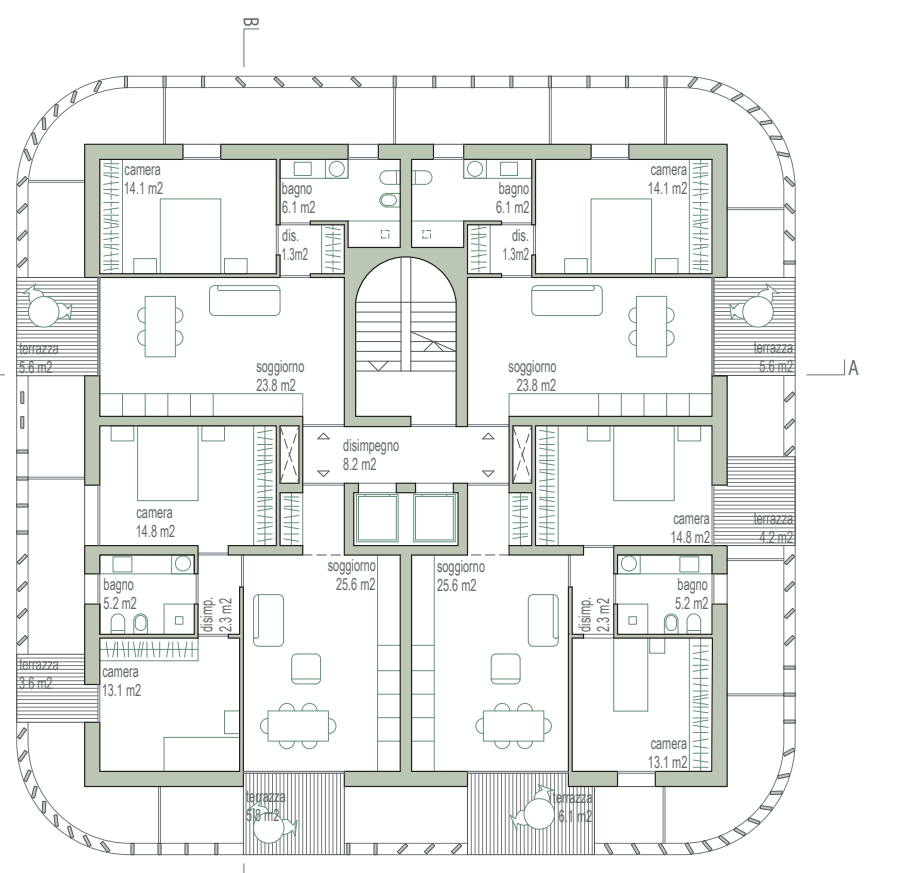
Tipologia 3 camere
