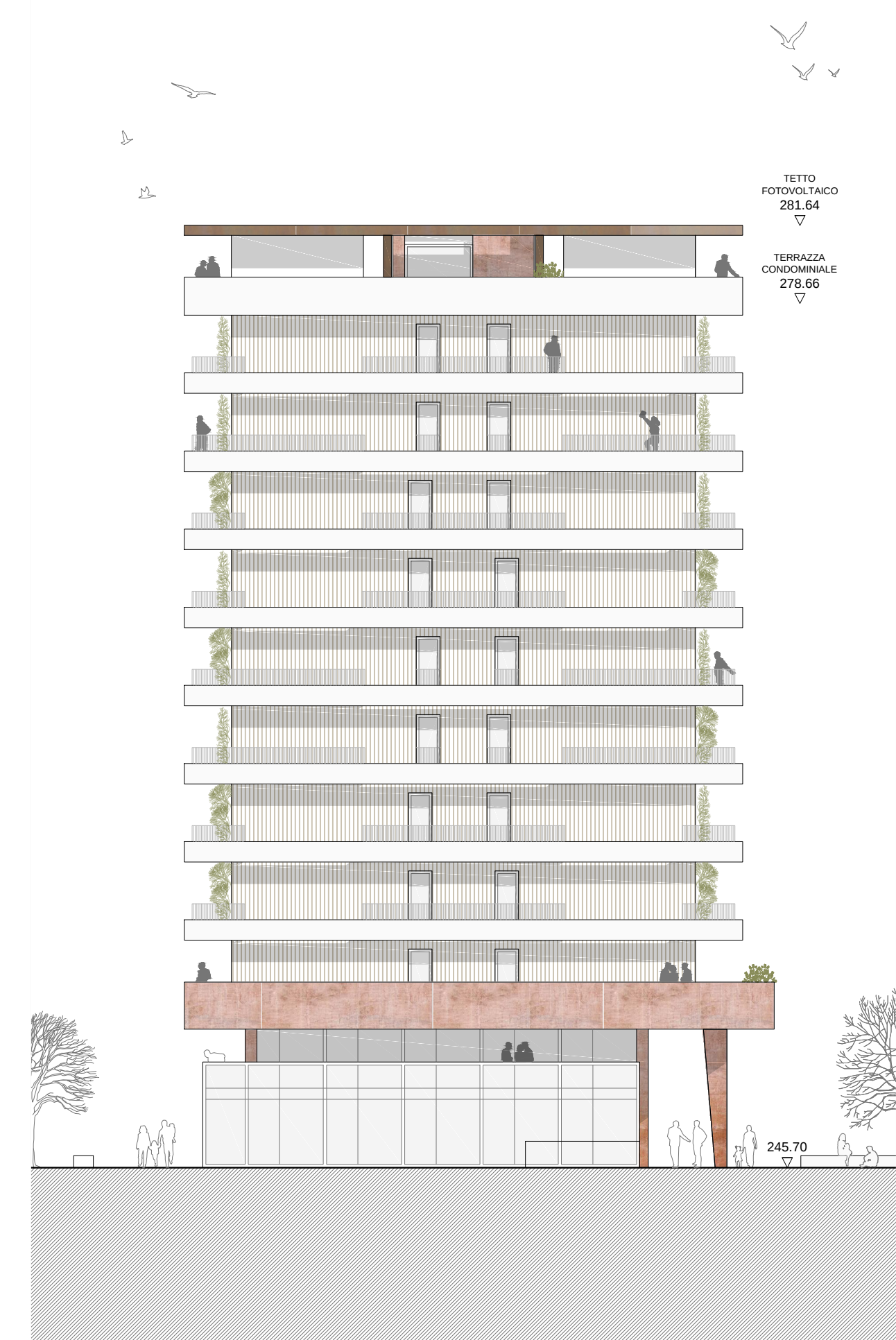
PROSPETTO NORD SCALA 1:200
