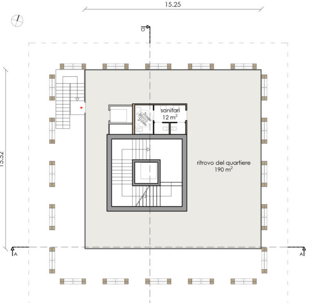
PIANO 1° SCALA 1:200
