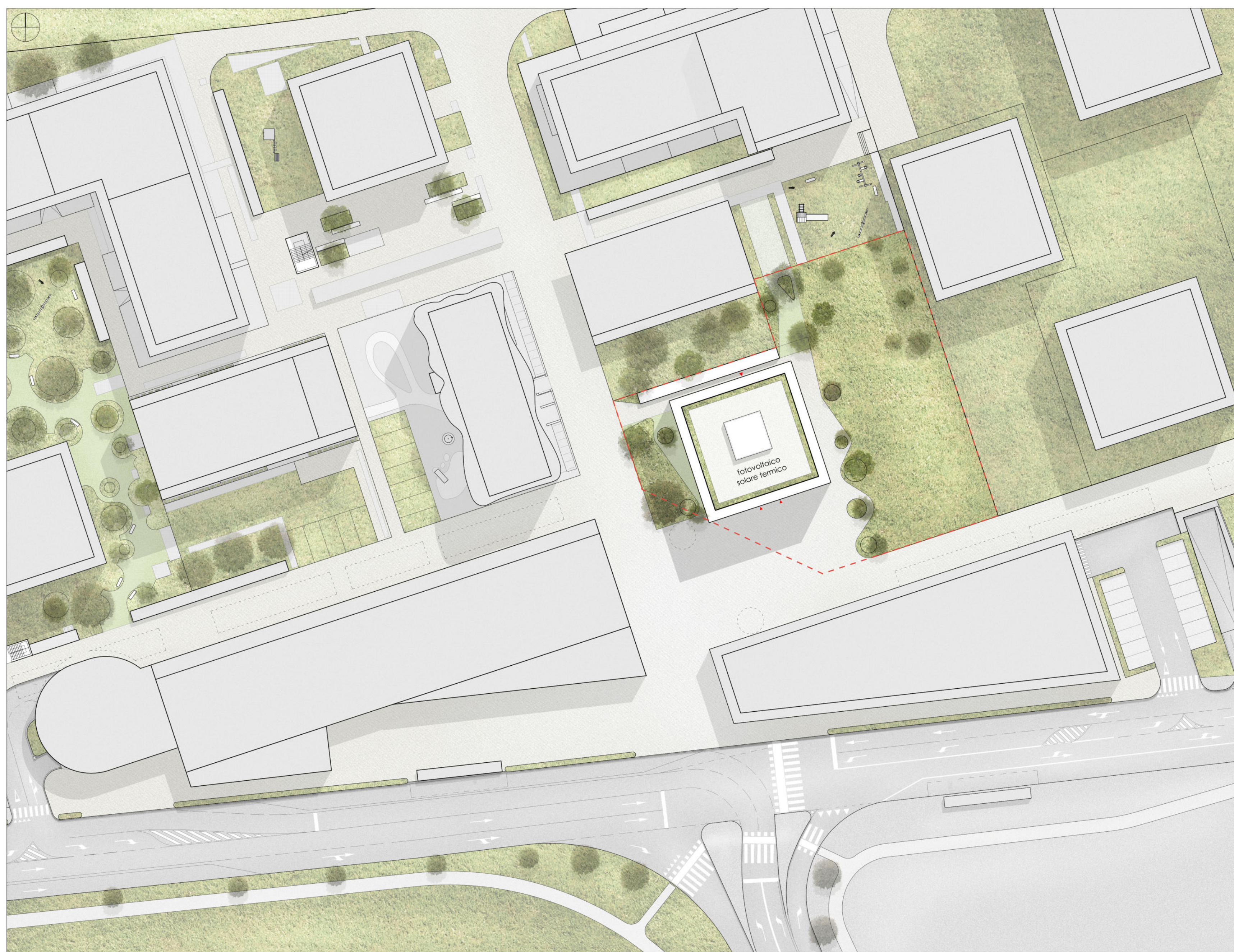
PLANIMETRIA SCALA 1:500
