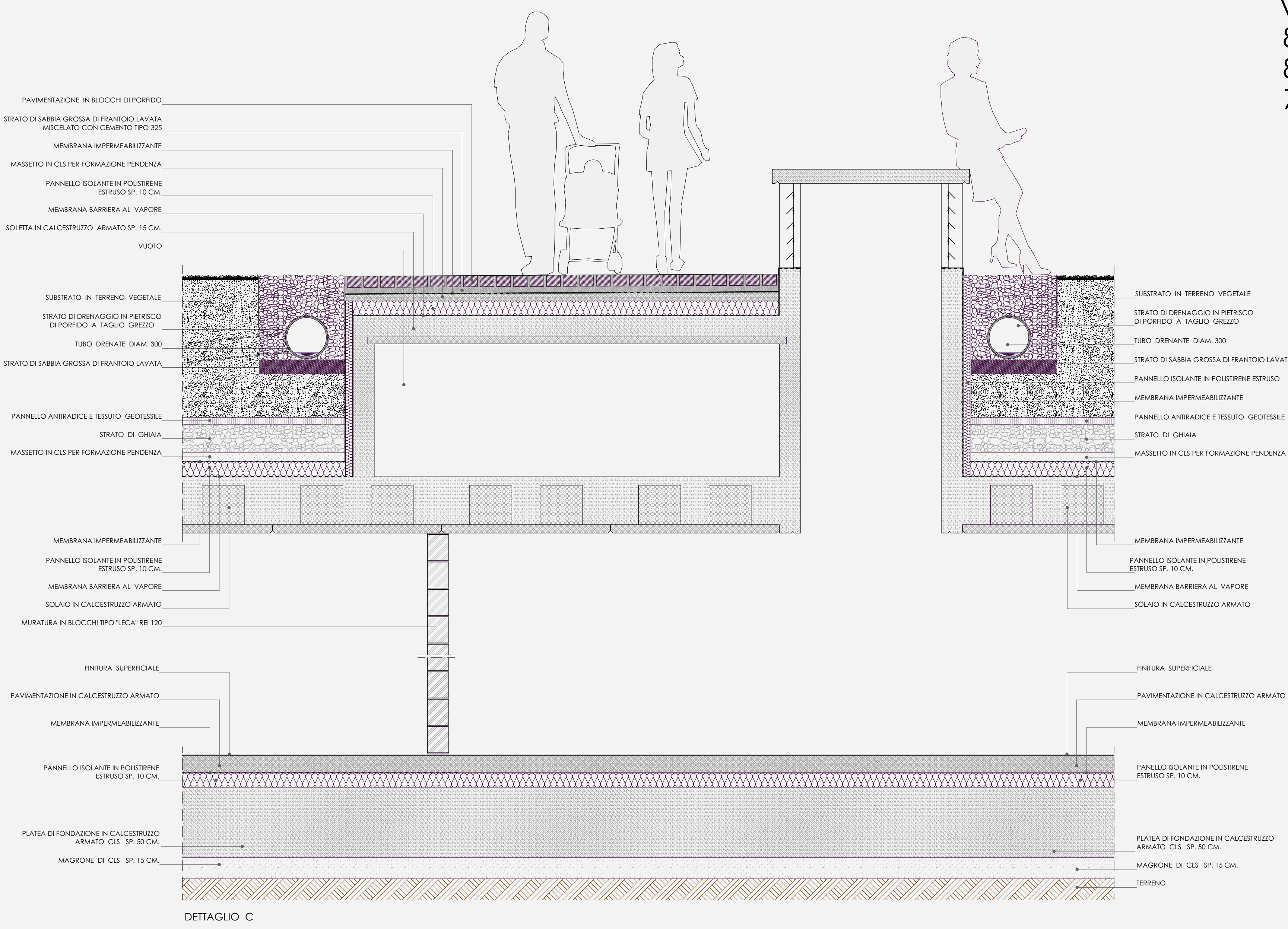
DETTAGLIO C
