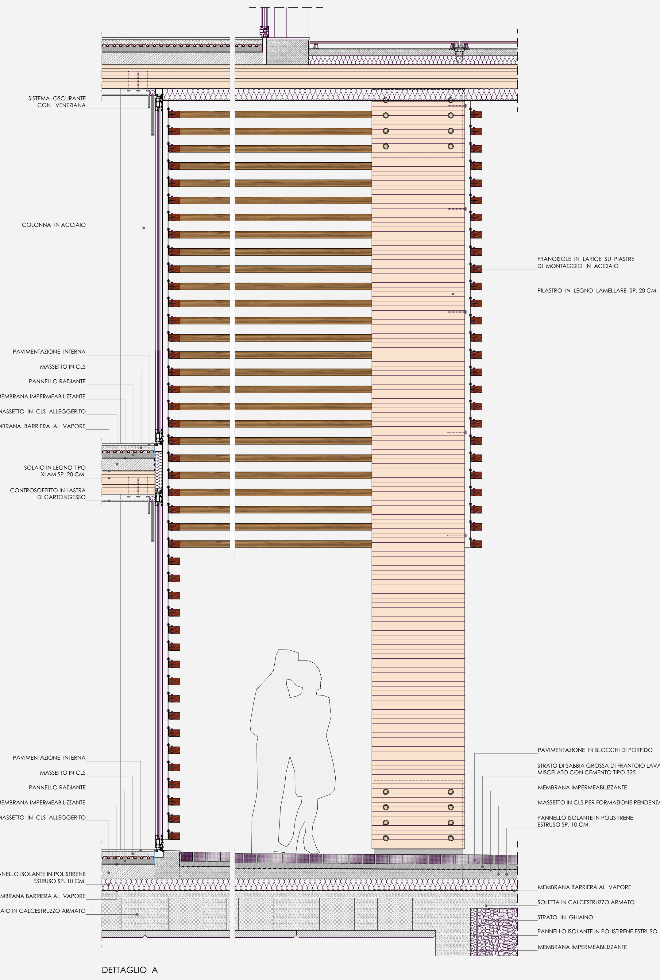
DETTAGLIO A
