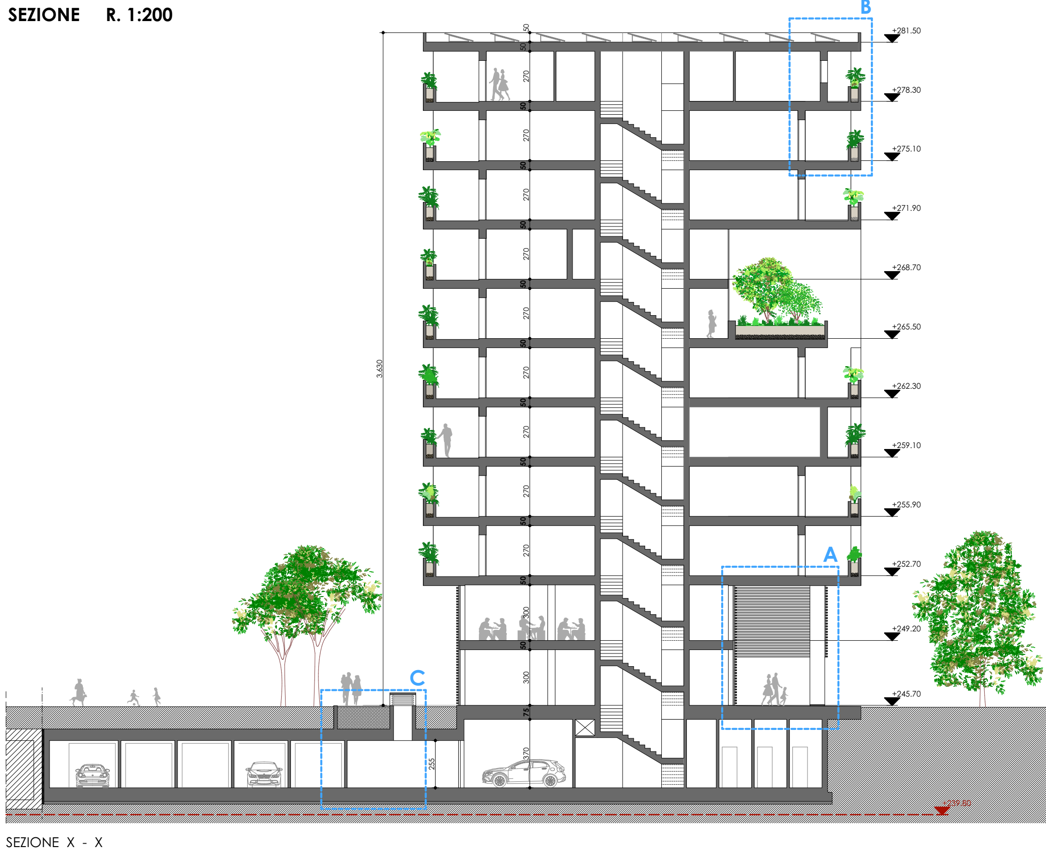
SEZIONE R. 1:200
