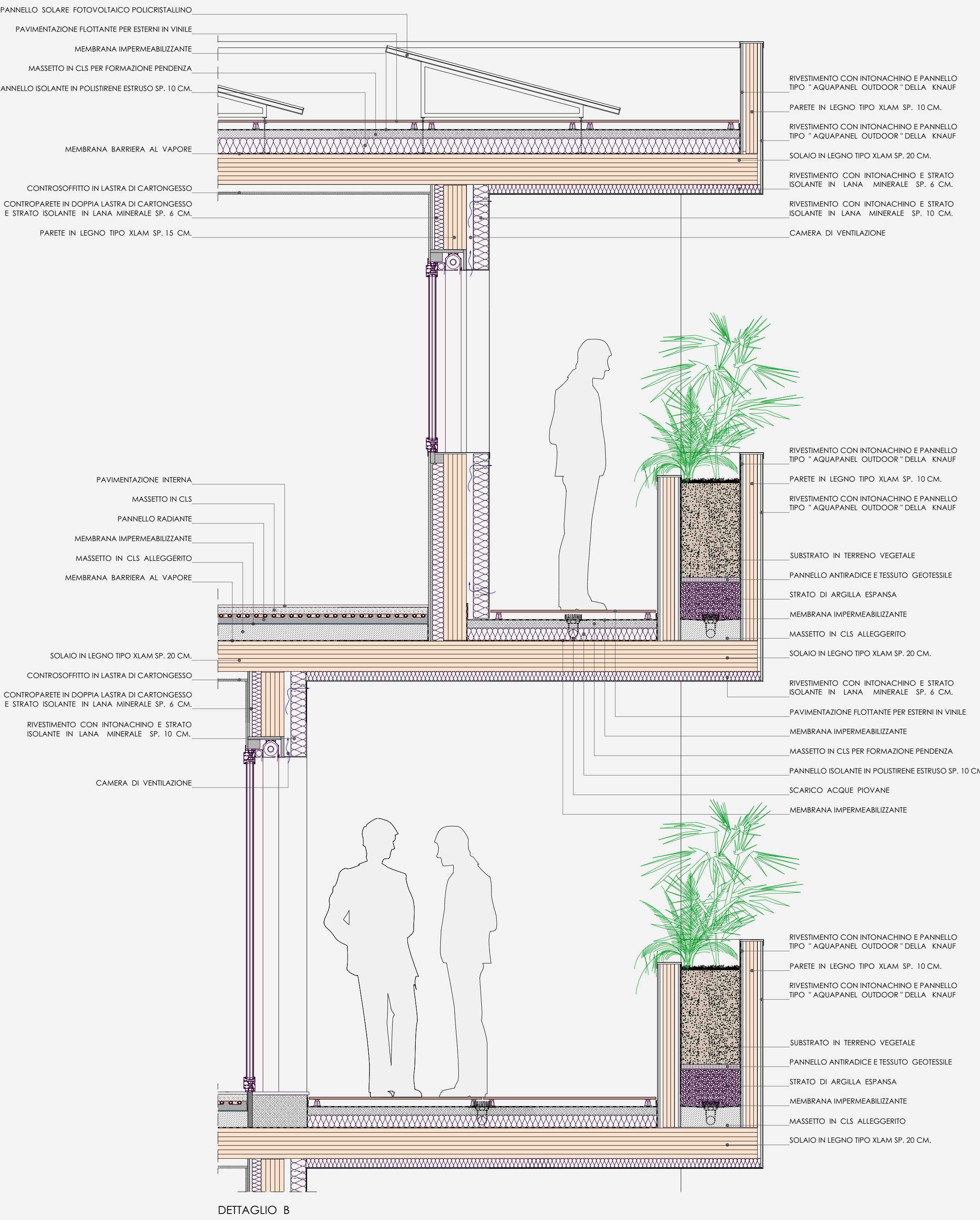
DETTAGLIO B
