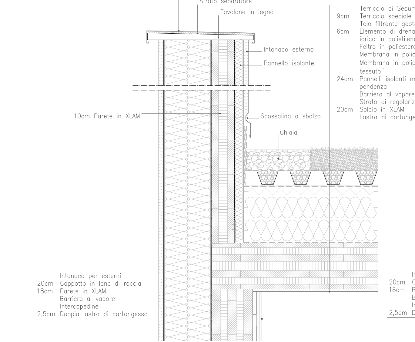
NODO SOLAIO DI COPERTURA SCALA 1:20
