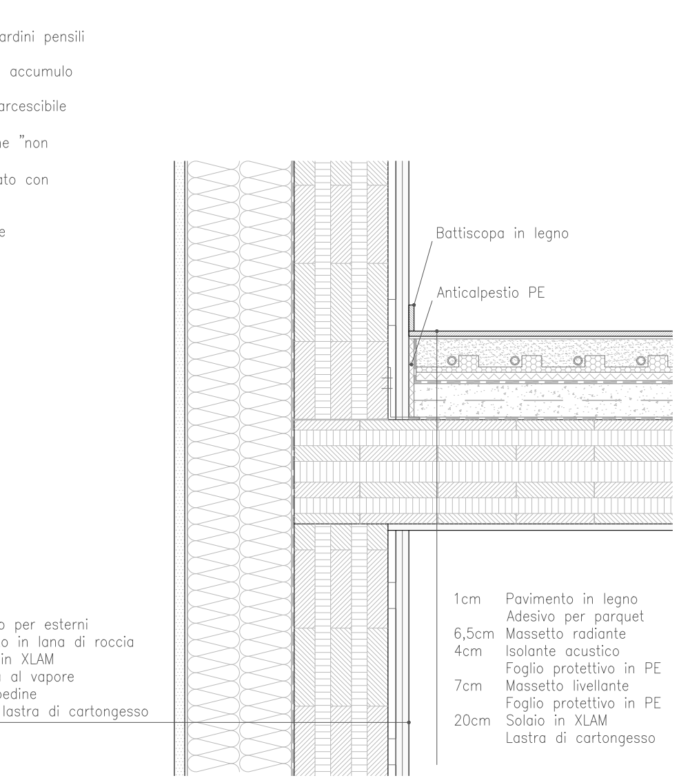
NODO SOLAIO INTERMEDIO SCALA 1:20
