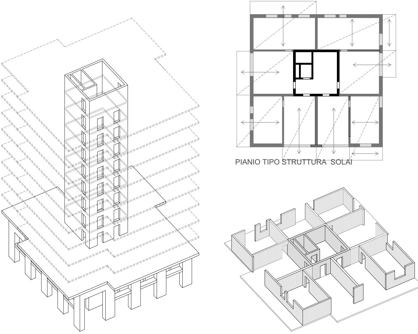
BASAMENTO E NUCLEO CENTRALE IN CLS
