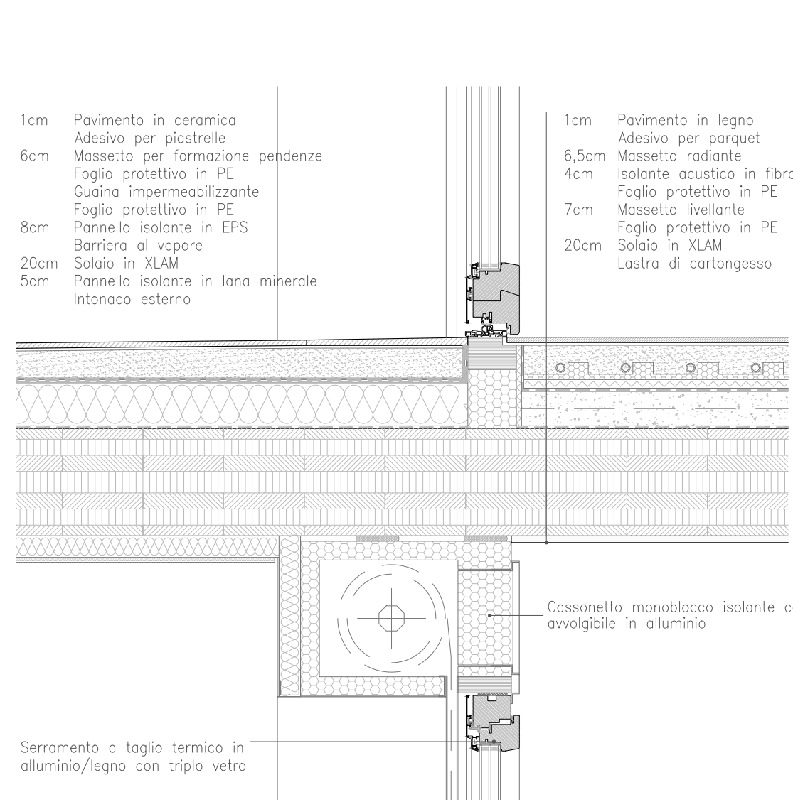
NODO BALCONE SCALA 1:20
