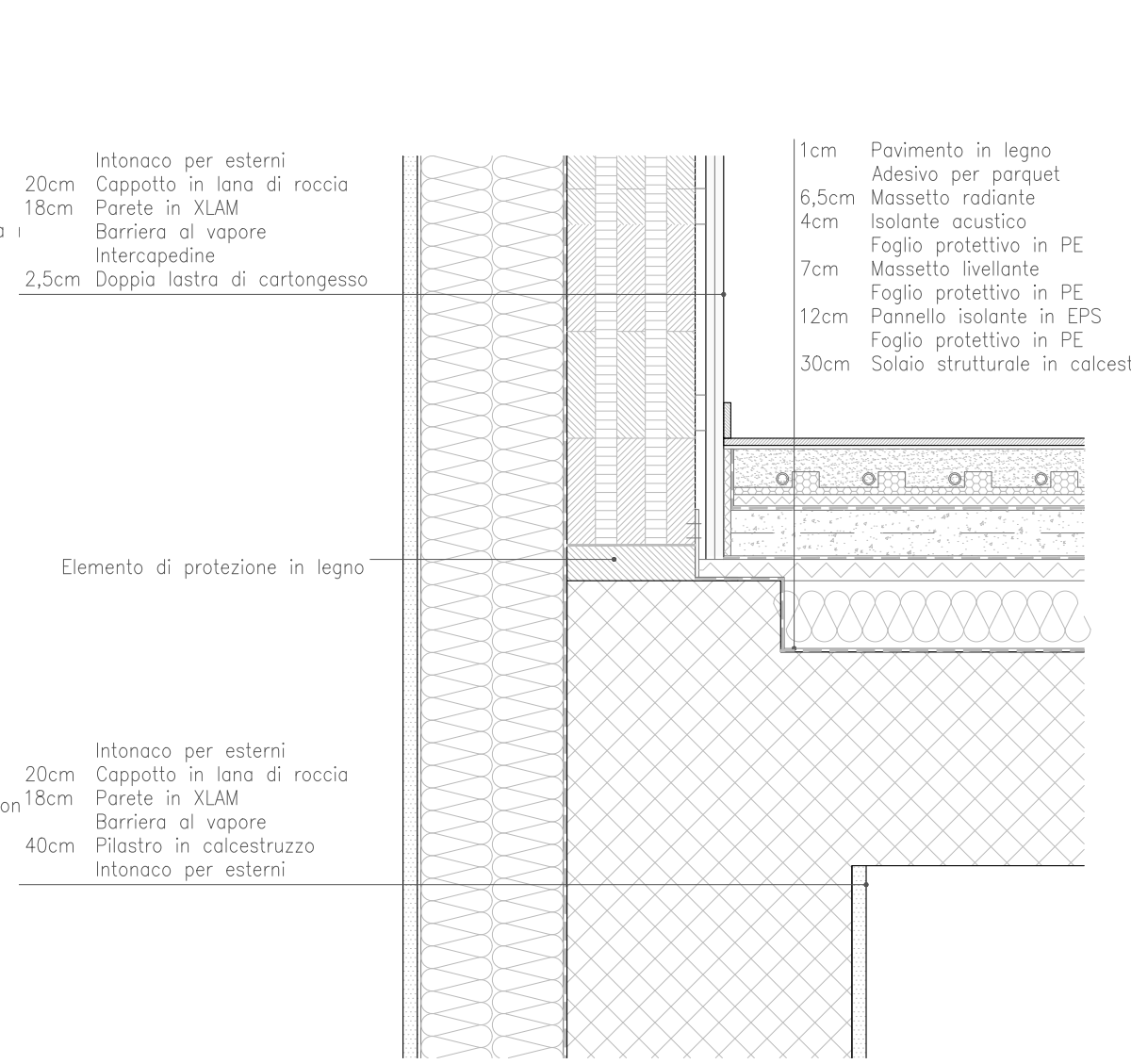
NODO SOLAIO PORTICO SCALA 1:20
