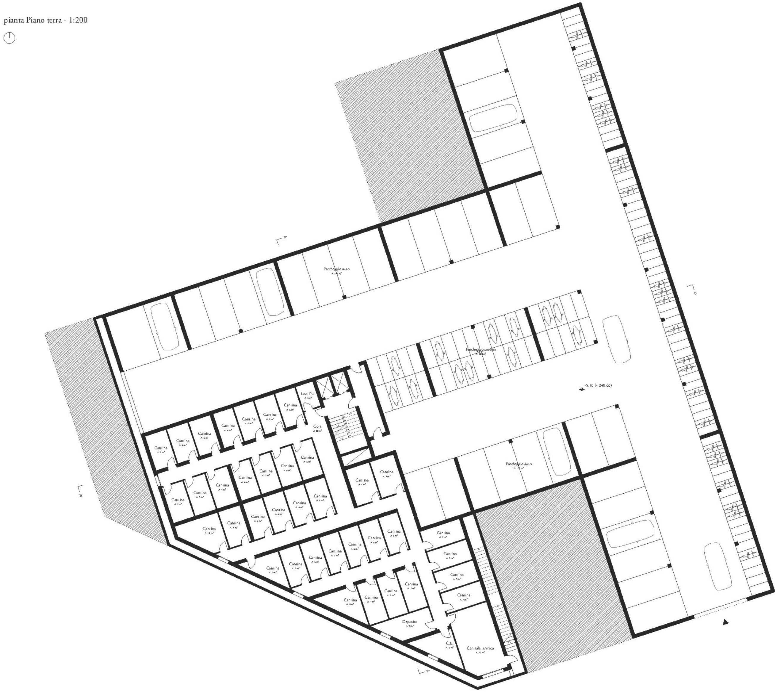
pianta Piano interrato - 1:200
