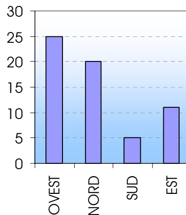
Distribuzione spaziale degli eventi
