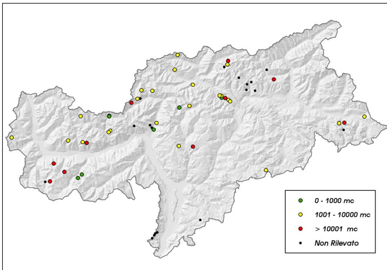
Rappresentazione distribuita dell'entità volumetrica degli eventi
