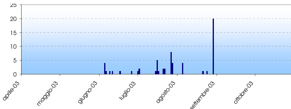
Distribuzione temporale in dettaglio
