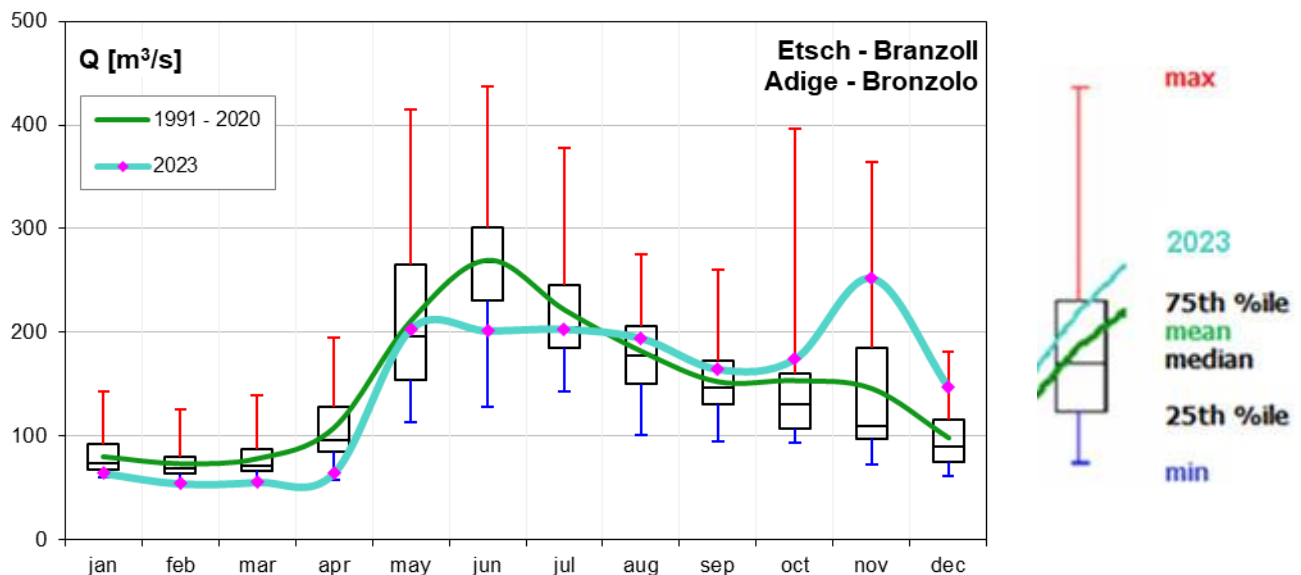
Abb 3.1. Vergleich der mittleren monatlichen Abflüsse ( Q_{\text{mean}} [ \text{m}^3/\text{s} ]) in der klimatologischen Referenzperiode 1991 – 2020 mit jenen von 2023 gemessen an der Pegelstation Etsch – Branzoll
