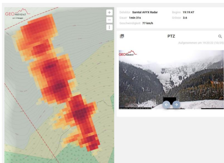
Abb. 6.4: Vom Lawinenradar erfasste Staublawine der Pichlereschbaumlawine in Weissenbach/Sarntal
