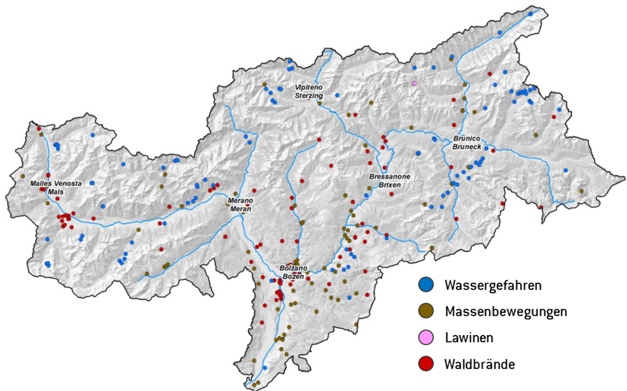
Abb 2.6: Geografische Verteilung der Naturereignisse im Jahr 2022 in Südtirol
