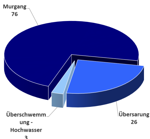
Grafiken 4.3 e 4.4: Klassifizierung der hydraulischen Ereignisse und der Schäden
