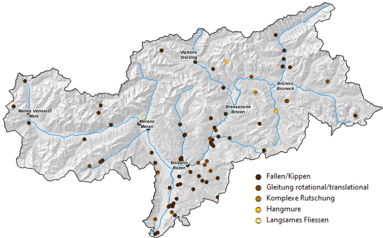
Abb 5.7: Geographische Verteilung der Massenbewegungen im Jahr 2022 in Südtirol
