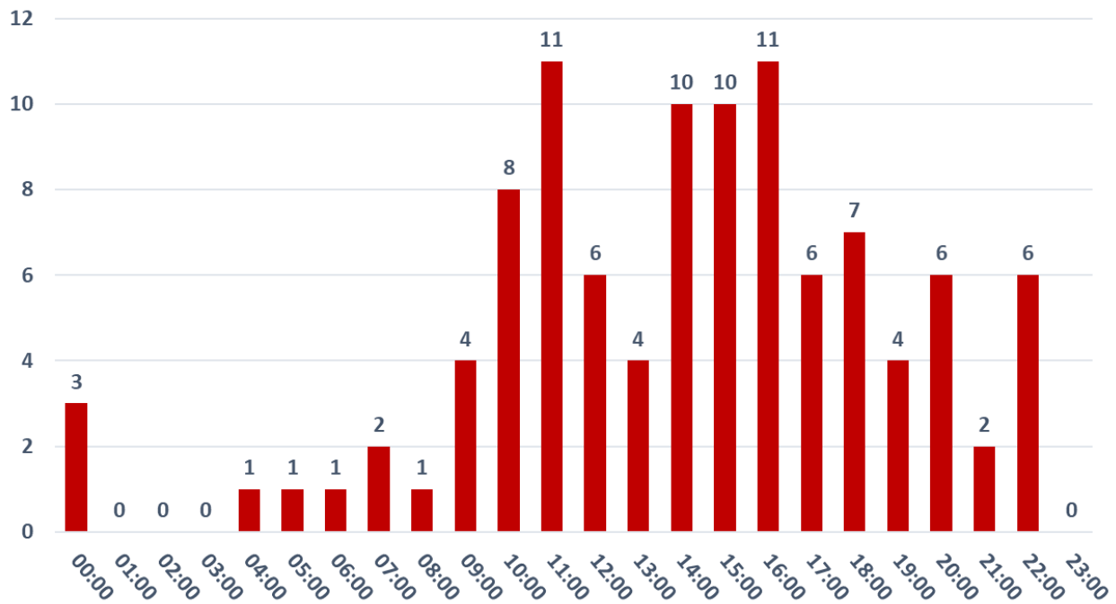
Grafik 7.8: Aufteilung der Waldbrände innerhalb der 24 Stunden – Jahr 2022
