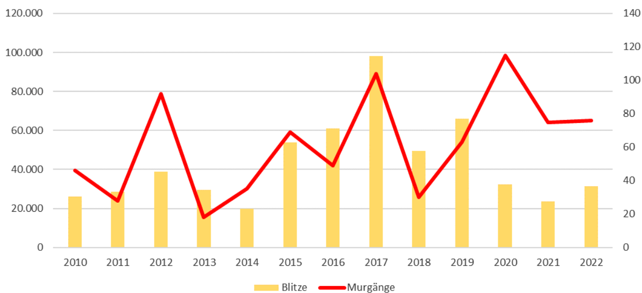
Grafik 4.6: Gegenüberstellung der Murereignisse mit den Blitzereignissen der Periode 2010-2022
