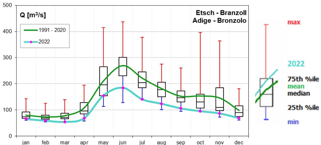
Abb. 3.1: Vergleich der mittleren monatlichen Abflüsse ( Q_{\text{mean}} [ \text{m}^3/\text{s} ]) in der klimatologischen Referenzperiode 1991 – 2020 mit jenen von 2022 gemessen an der Pegelstation Etsch – Branzoll
