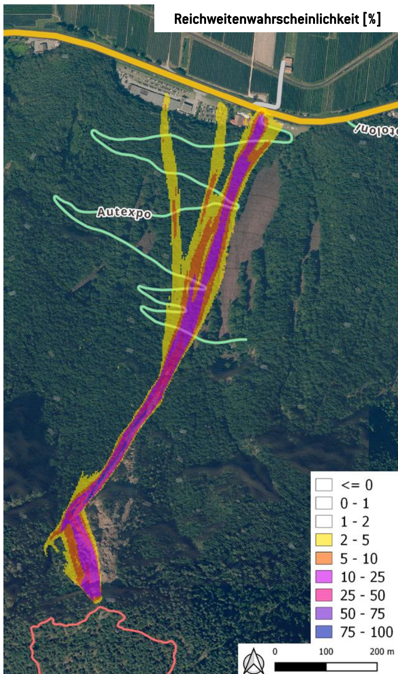
Abb. 5.10: Wahrscheinlichkeit der Reichweite der durchgeführten Steinschlagsimulationen. Die Ergebnisse spiegeln sehr gut das eingetretene Ereignis wider, wie die hohe Wahrscheinlichkeit von 10 – 25 % im Bereich der Pizzeria zeigt.
