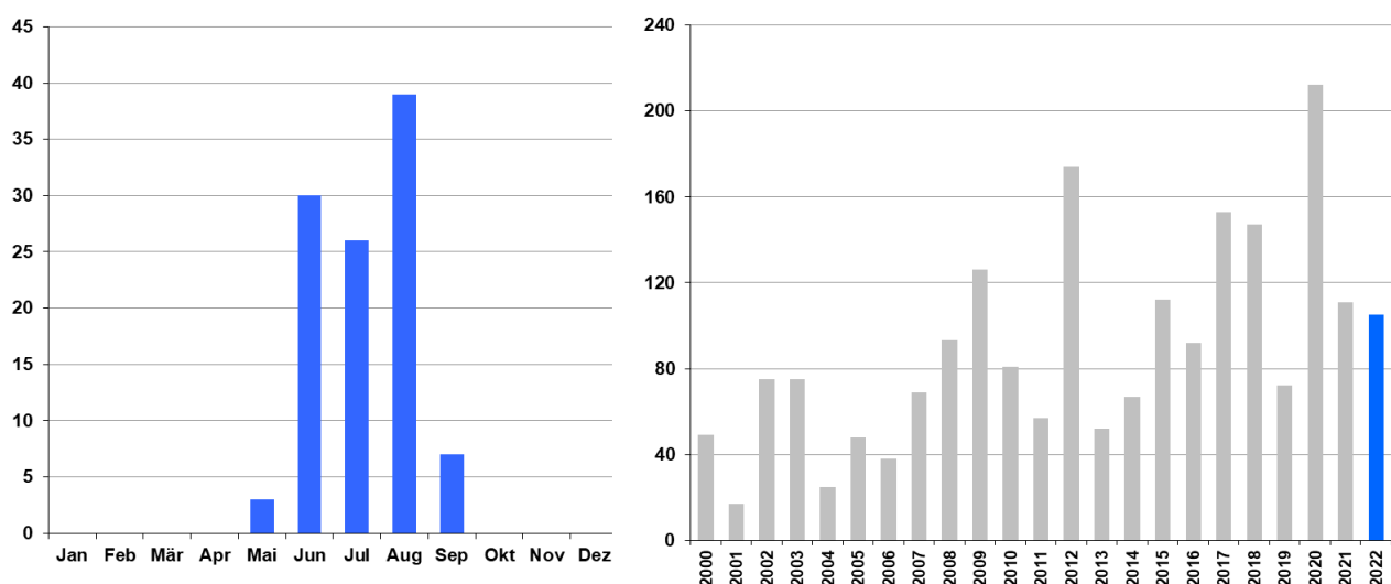
Grafiken 4.1 e 4.2: Zeitliche Verteilung der erhobenen hydraulischen Ereignisse 2022 und im Zeitraum 2000-2022
