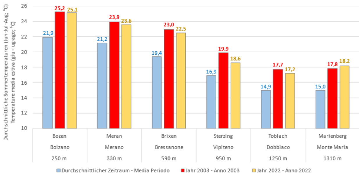
Grafik 7.4: Vergleich der durchschnittlichen Sommertemperatur im Jahr 2003, 2022 und der durchschnittlichen Temperatur über den gesamten Zeitraum der verfügbaren historischen Reihen
