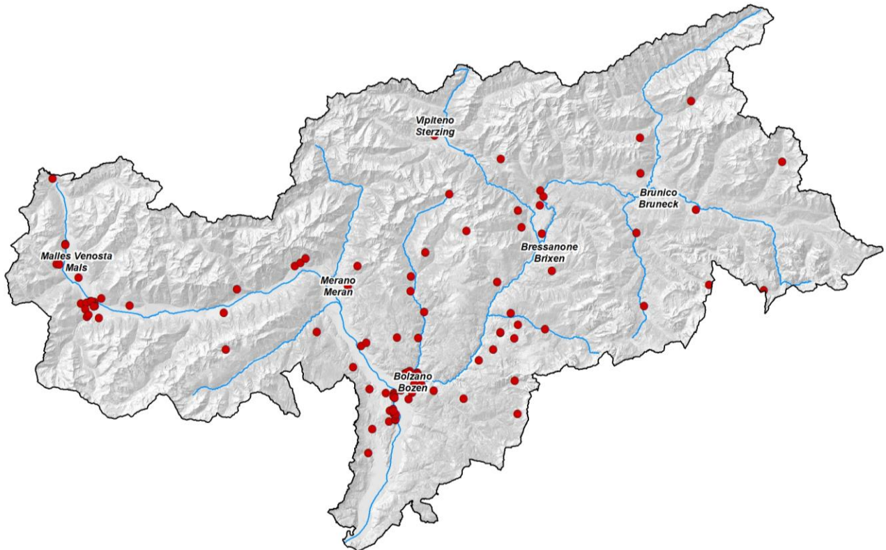
Abb. 7.3: Geographische Verteilung der Walbrände 2022 in Südtirol
