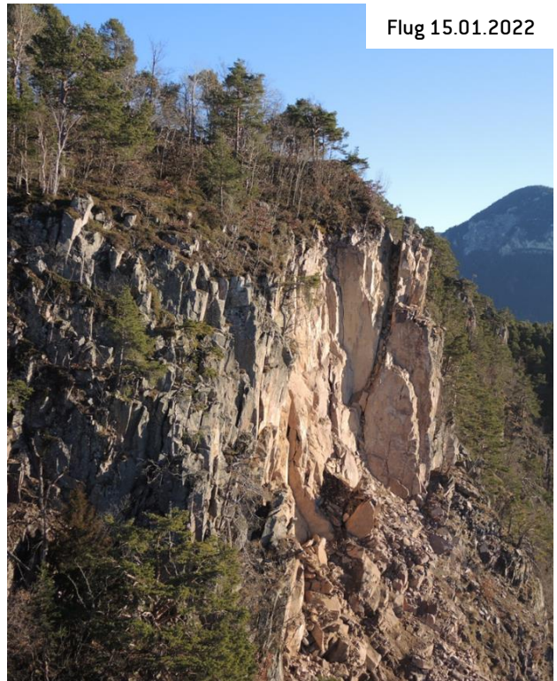
Abb. 5.9: Fotovergleich der Abbruchnischen des Felssturzes 2018 und 2022, anhand unterschiedlicher Flugaufnahmen. Sowohl in der Frontal- als auch in der Lateralansicht kann man das Abbruchvolumen vom 15. Jänner 2022 sehr gut eingrenzen.
