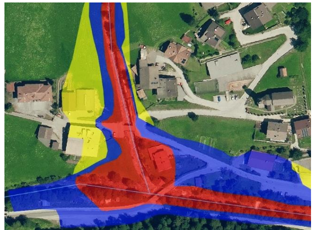
Abb. 4.14: Naturereignisse sind als Hauptmaßstab für Plausibilitätsprüfungen der Gefahrenzonenpläne heranzuziehen. In diesem Fall entsprechen die im Gefahrenzonenplan ausgewiesenen Gefahrenzonen des Kogbaches exakt jenem Ereignis, das sich am 5. August ereignet hat.
