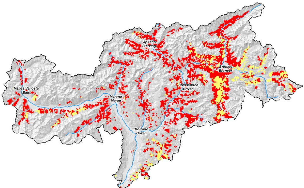
Abb 2.7: Geografische Verteilung der von Borkenkäfern betroffenen Gebiete; 2021 (Gelb) – 2022 (Rot)
