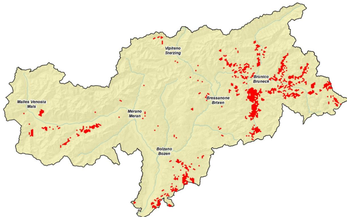
Abb 8.1: Geografische Verteilung der von Borkenkäfern im Jahr 2021 betroffenen Gebiete
