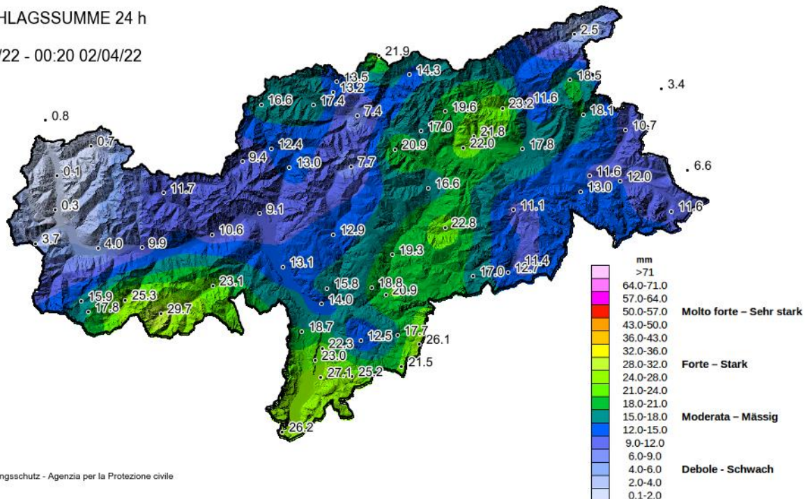
Abb. 6.3: Geografische Verteilung der Niederschlagssumme vom 2. April 2022.
