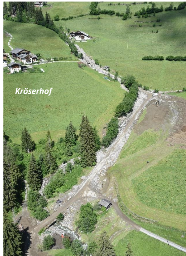
Abb 4.7: Wo ein loses, nicht verfestigtes (unkonsolidiertes) Bachbett vorhanden ist, können Hochwasserereignisse zu umfangreichen Erosionen führen. Konsolidierte Bachbetten sind allerdings oft unzureichend dimensioniert, insbesondere an Kreuzungspunkten, wie auf dem Foto unten links zu sehen ist.
