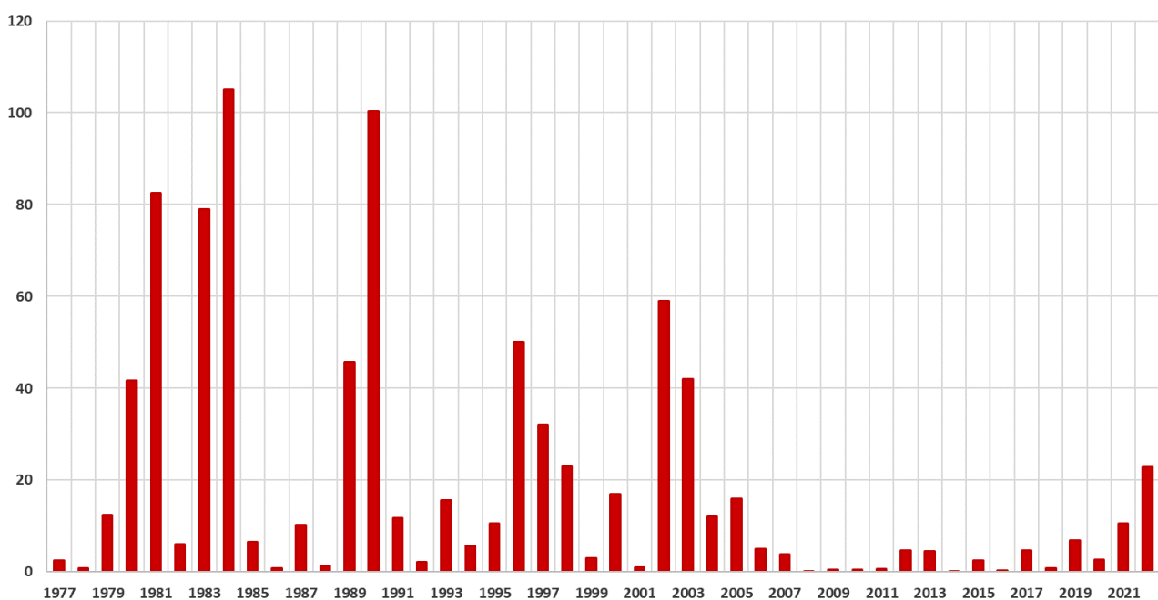
Grafik 7.7: Abgebrannte Fläche (ha) pro Jahr – Zeitraum 1977 – 2022
