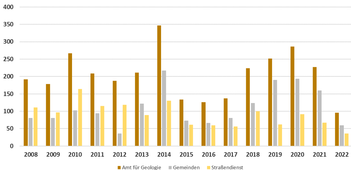
Grafik 5.3: Zeitreihe der Einsätze des Amtes für Geologie von 2008 bis 2022
