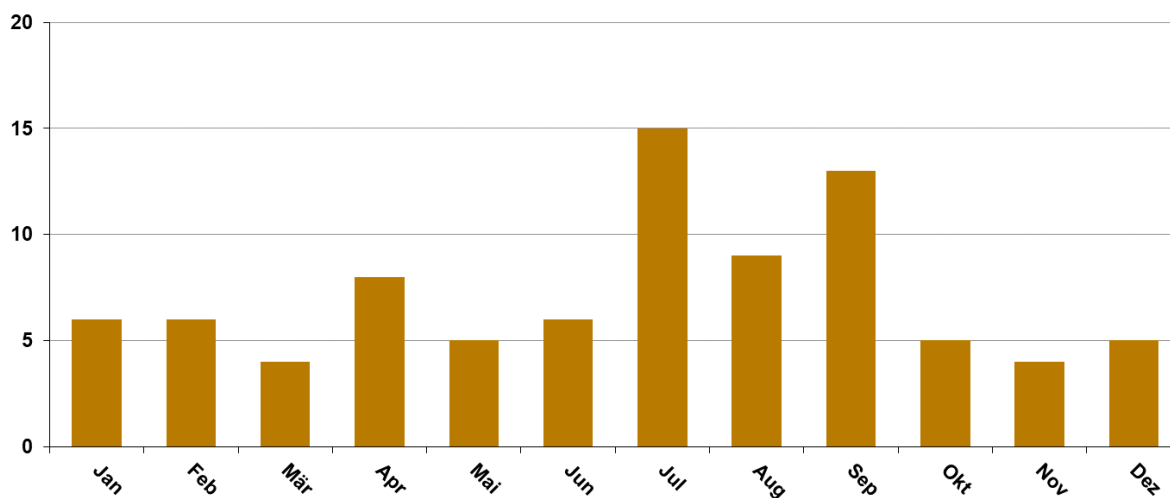
Grafik 5.1: Chronologische Verteilung der Massenbewegungen des Jahres 2022
