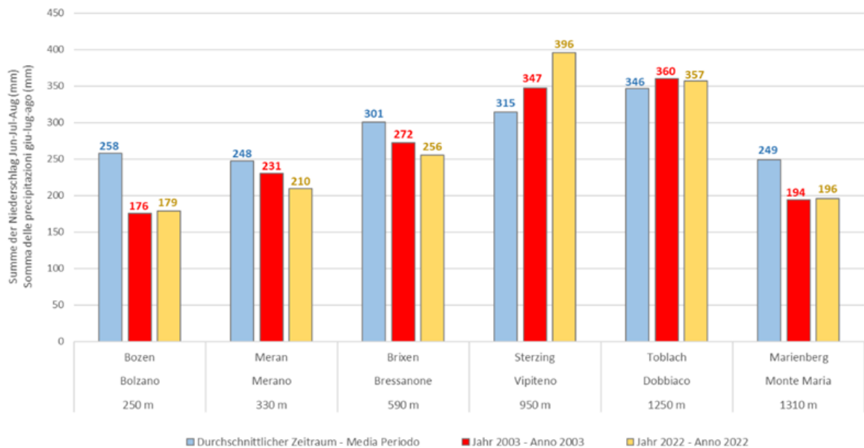
Grafik 7.5: Niederschlag im Sommer – Vergleich zwischen dem Durchschnitt für den Zeitraum 2003 und 2022
