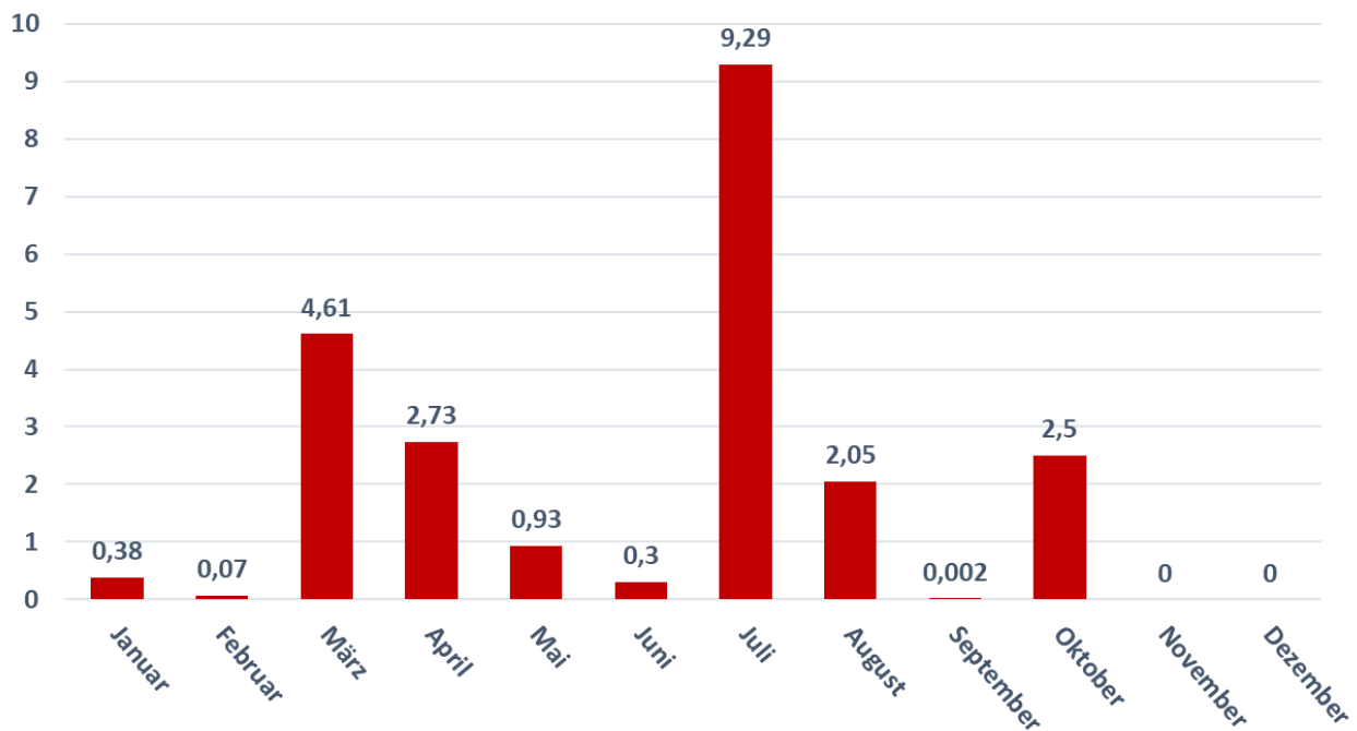
Grafik 7.9: Waldbrannfläche [ha] pro Monat – Jahr 2022
