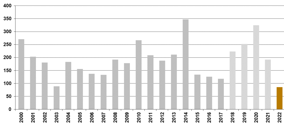
Grafik 5.2: Zeitreihe der Einsätze des Amtes für Geologie von 2000 bis 2022
