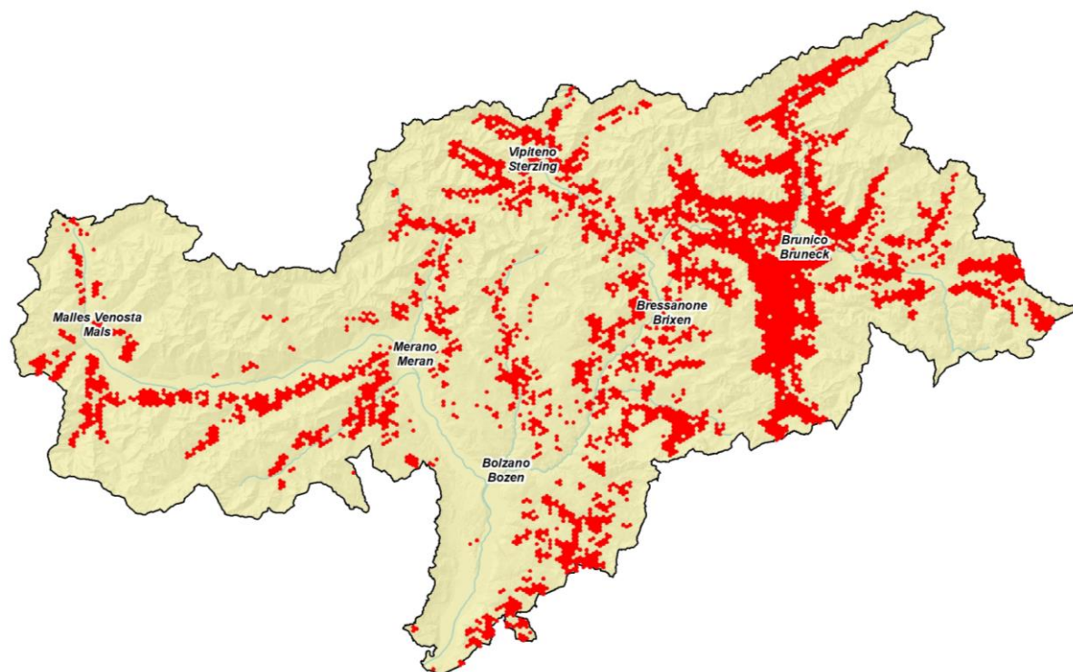
Abb 8.1: Geografische Verteilung der von Borkenkäfern im Jahr 2022 betroffenen Gebiete
