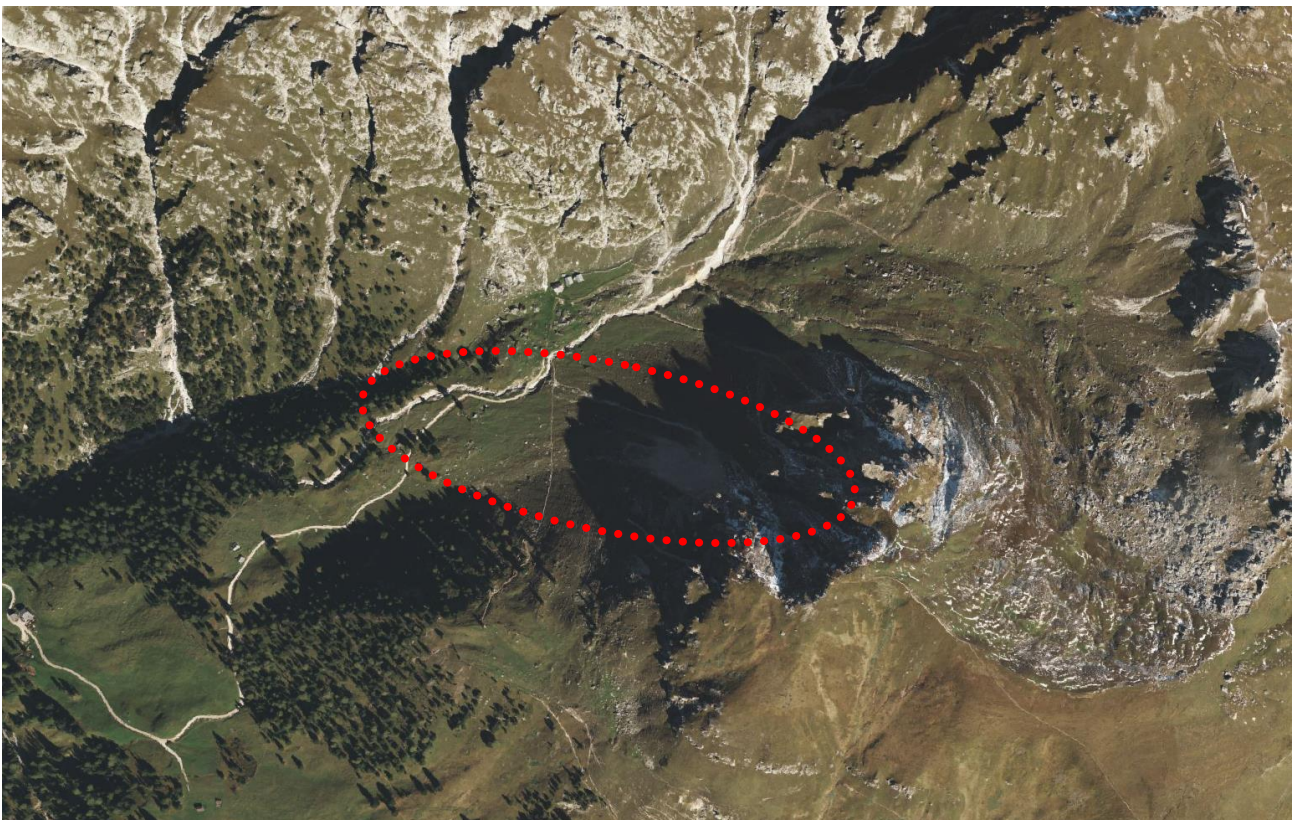
Abb. 5.12: Bing Luftbild 2023; der Ablagerungsbereich des Felssturzes ist deutlich erkennbar.
