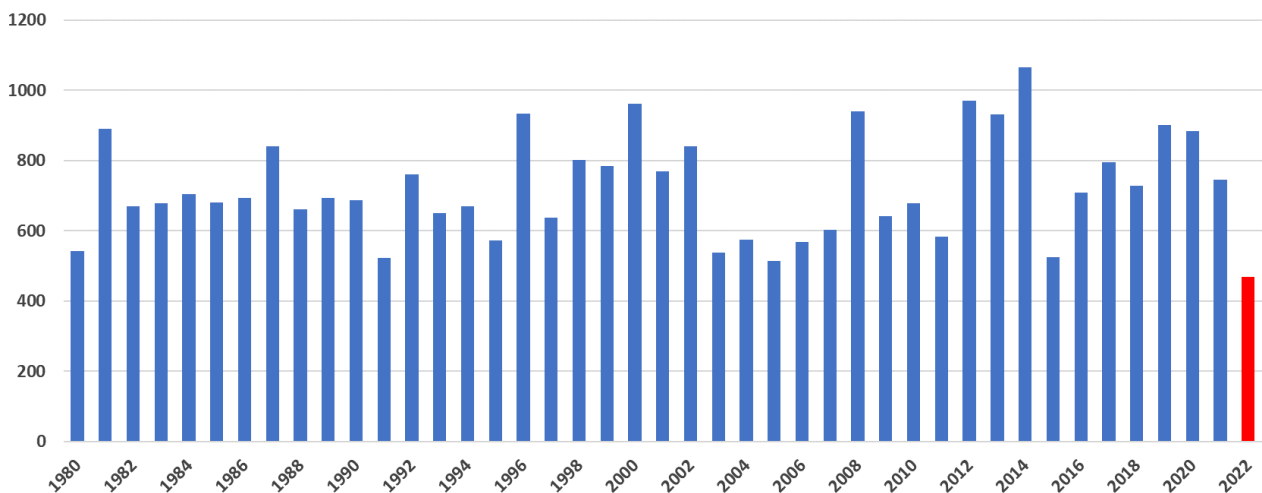
Grafik 2.3: Niederschläge an der Wetterstation Bozen (1980 – 2022)
