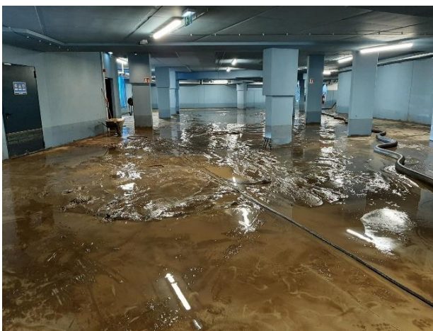
Abb. 4.9: a Das linke Bild zeigt die Überflutung der Tiefgarage des Hotels Lido, die den Einsatz der Freiwilligen Feuerwehr erforderte. Selbst kleine Wassermengen können, wenn sie Eintrittsstellen finden, in Kellerräumen große Schäden verursachen, insbesondere an Fahrzeugen und technischen Anlagen. Rechts: Schutt- und Geröllablagerungen im Gartenbereich.
