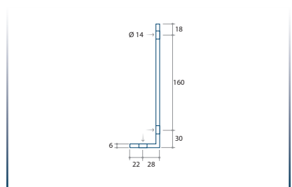
E200 - Befestigungsplatte für Sigma Profile
