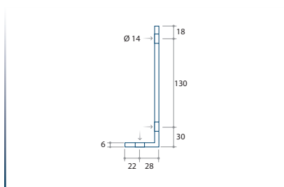
E170 - Befestigungsplatte für Sigma Profile
