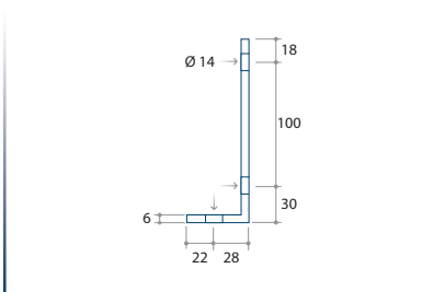
E140 - Befestigungsplatte für Sigma Profile
