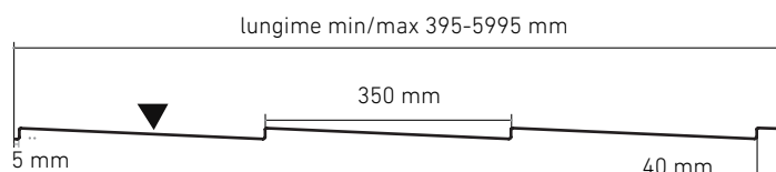
SECȚIUNE LOGITUDINALĂ
