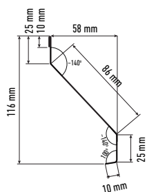
Profil jaluzeala tip L
