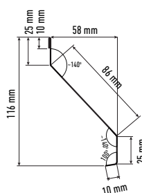
Profil cadru gard tip jaluzeala D
