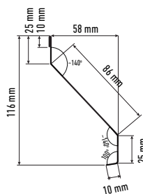
Profil cadru gard tip jaluzeala L
