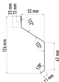
Profil jaluzeala tip D
