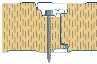
Verborgen bevestiging
