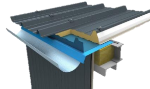
Dachrinnen
