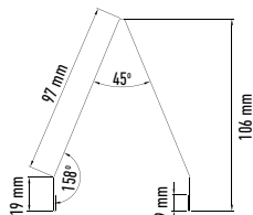
Profil jaluzele tip A
