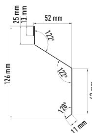
Profil jaluzele tip D
