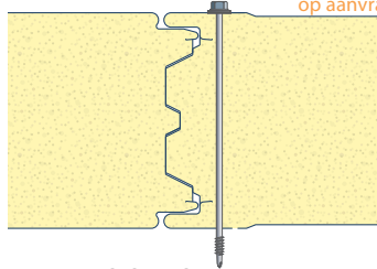
Zichtbare bevestiging driedubbele sluiting
