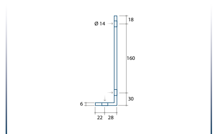
E200 - Befestigungsplatte für Sigma Profile
