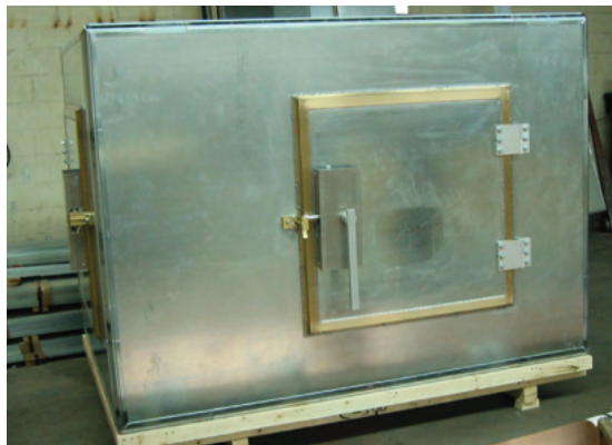
RFID Test Box
